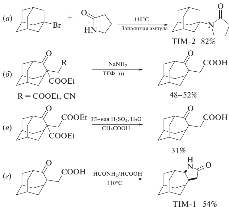
Рис. 1. Схемы синтеза соединений. Синтез 1-(адамантан-1-ил)пирролидин-2-она (ТИМ-2) (а); синтез 2-(5-оксотрицикло[4.3.1.1 3,8 ]ундекан-4-ил)уксусной кислоты по реакции Холлера–Бауэра (б); гидролиз-декарбоксилирование этил-4-(2-этоксикарбонилметил)-5-оксотрицикло[4.3.1.1 3,8 ]ундекан-4-карбоксилата (в); синтез (3а5*,10а5*)-декагидро-4,8:6,10-диметаноциклононан[б]пиррол-2(1H)-она (ТИМ-1) (г).
