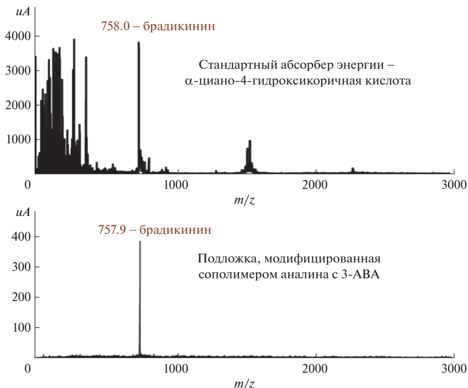
Рис. 6. Определение брадикинина методом SELDI-TOF-MS на кремниевых чипах, модифицированных сополимером 3-АВА-РАНИ (адаптированный рисунок из патента Vaczine-Shlosser et al. [45]).
