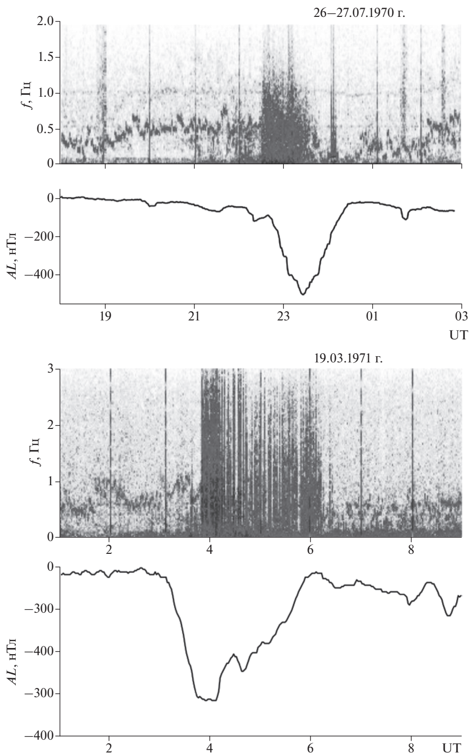
Рис. 1. Типичные примеры нарушения режима генерации “серпентинной эмиссии” в обл. Восток во время развития изолированных суббури в авроральном овале: (а) – 26–27.07.1970 г., (б) – 19.03.1971 г. В верхней части рисунков представлены динамические спектры УНЧ-колебаний, внизу – вариации AL -индекса.
