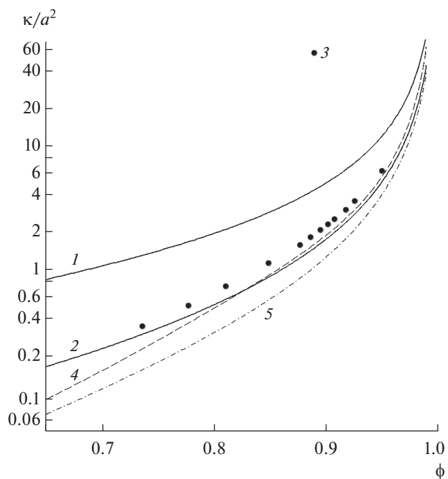
Рис. 8. Зависимости проницаемости \kappa a^{-2} от пористости \phi = 1 - \alpha , 1, 2 – прямое численное моделирование для ДГМ 3D-фильтра при \text{Kn} = 1 (1) и \text{Kn} = 0 (2), 3 – расчеты для неоднородных рядов волокон [24], 4 – по эмпирической формуле Девиса (16), 5 – по формуле Кувабары для ячеечной модели с 2D полем течения.
