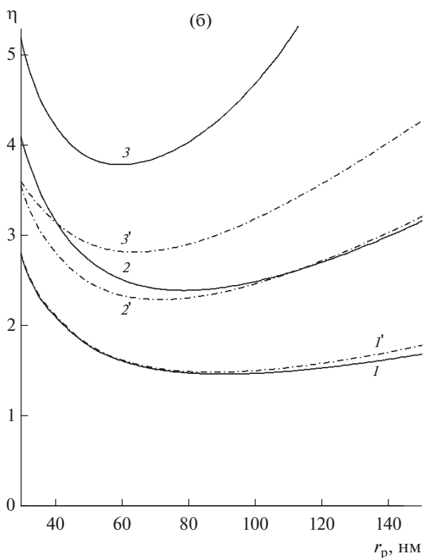
Рис. 7. Зависимости коэффициента захвата от радиуса частиц: (а) a = 100 нм, (б) a = 50 нм; b = 0.01 (1, 1'), b = 0.1 (2, 2'), b = 0.2 (3, 3'). 1'–3' – ряд параллельных волокон (2D), 1–3 – ДГМ 3D-фильтр, U = 2 см/с.
