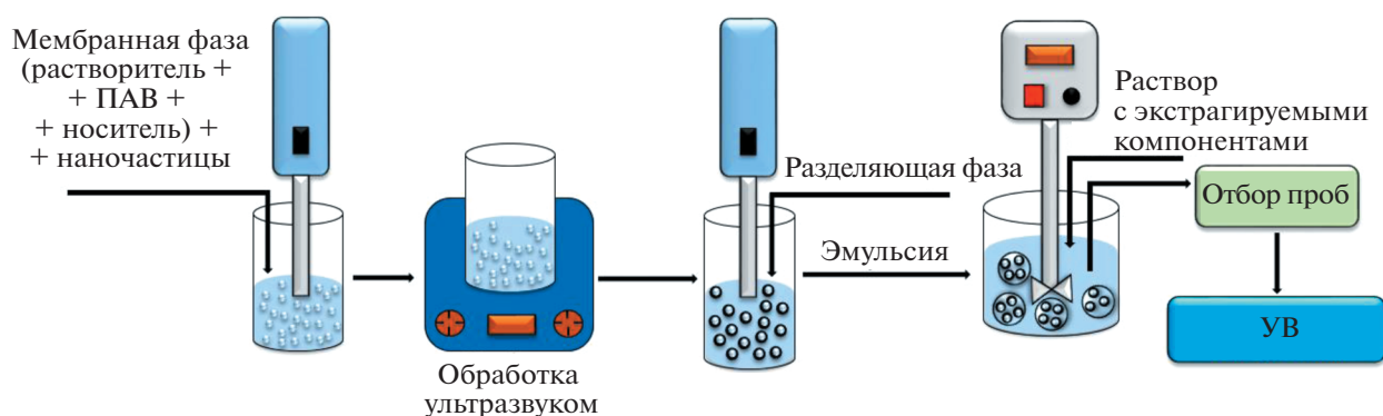
Рис. 1. Схематическое представление работы эмульсионной наножидкостной мембранной системы.
