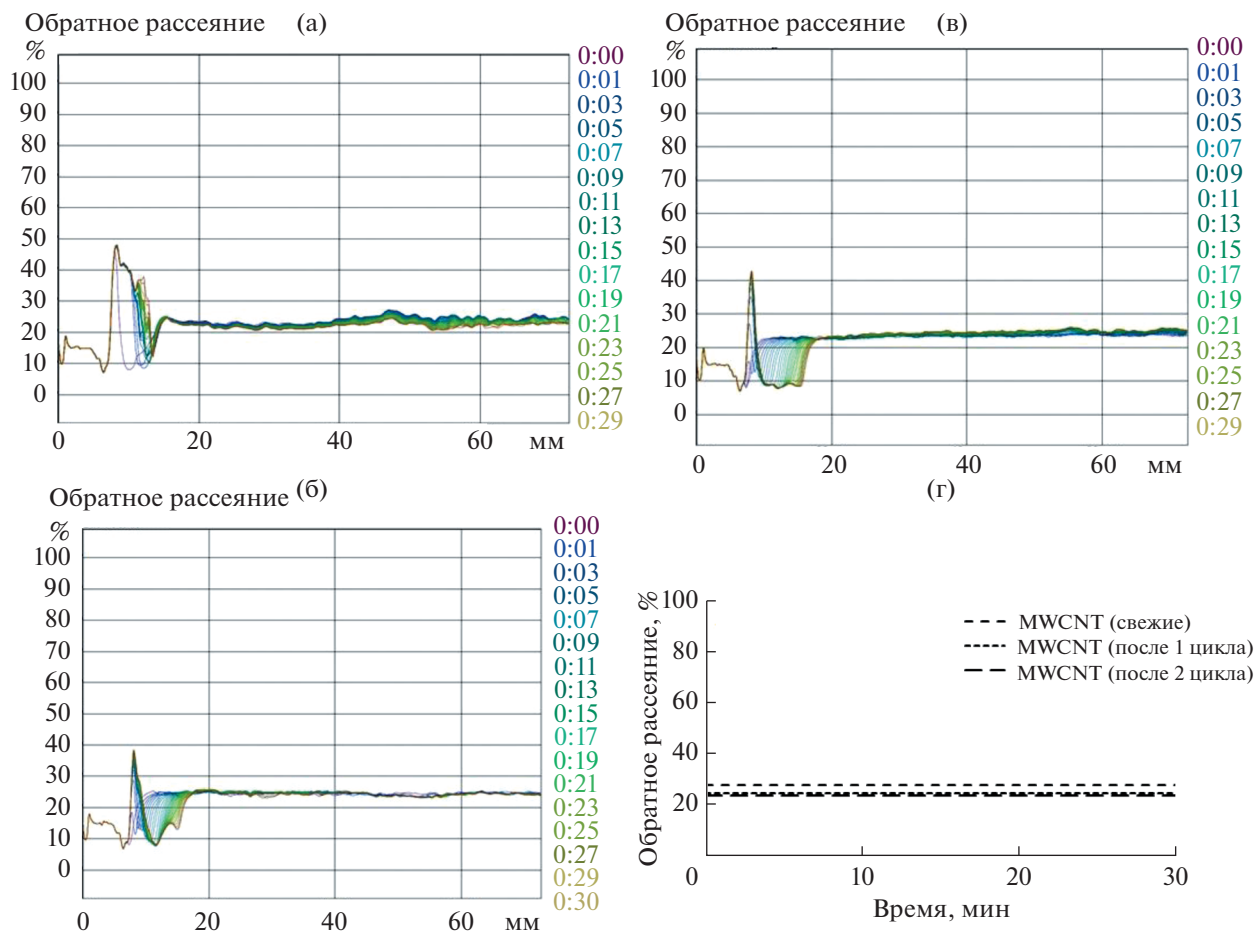
Рис. 8. Профили обратного рассеяния эмульсии, содержащей MWCNT: (а) цикл 1; (б) цикл 2; (в) цикл 3; (г) средние профили обратного рассеяния эмульсий, содержащих MWCNT.
