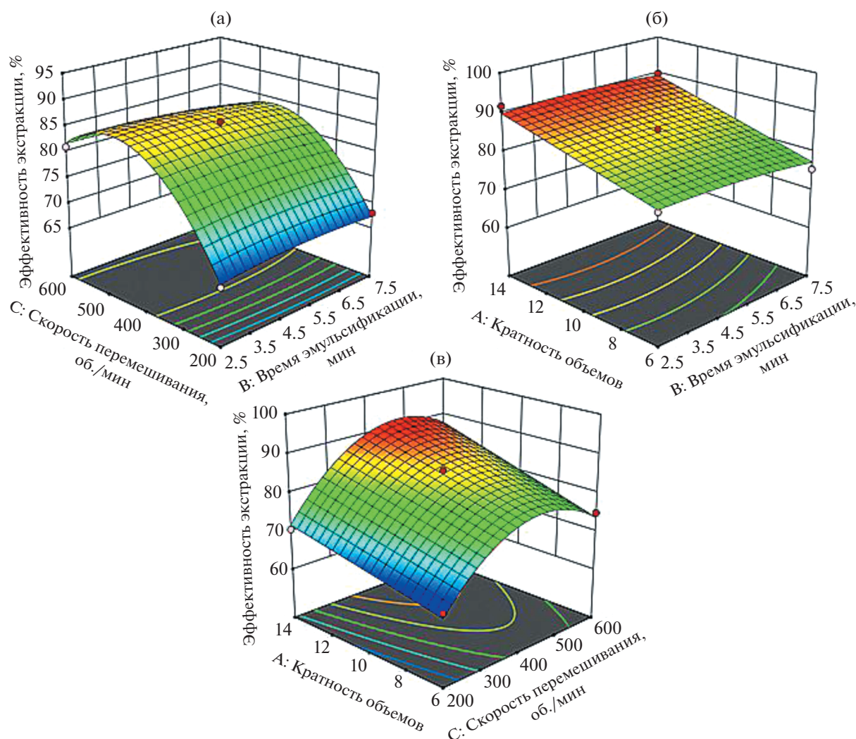
Рис. 3. Трехмерные графики поверхности отклика для эффективности экстракции (%) диклофенака в зависимости от (а) времени эмульгирования и скорости перемешивания; (б) времени эмульгирования и кратности объемов; (в) скорости перемешивания и кратности объемов.
