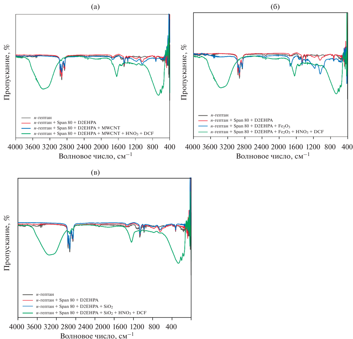
Рис. 4. ИК-спектры нарушенного полного отражения мембранной фазы до и после экстракции: (а) MWCNT; (б) \text{Fe}_2\text{O}_3 ; (в) \text{SiO}_2 .
