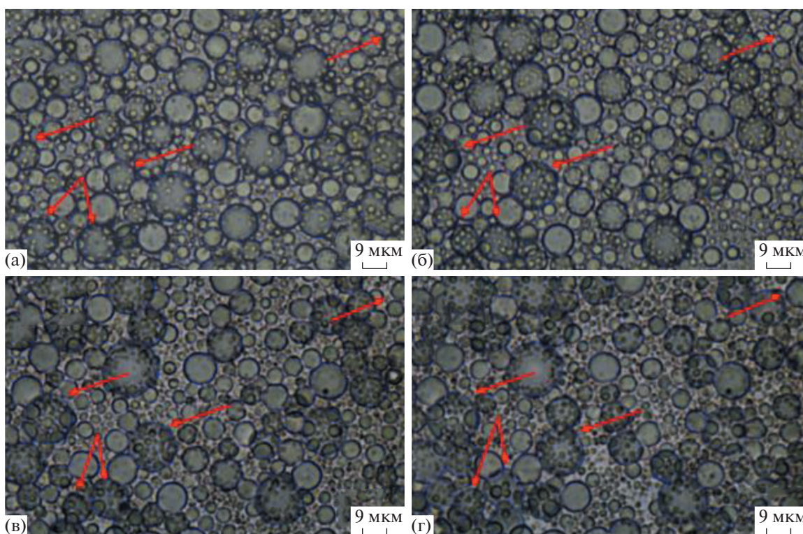
Рис. 11. Микрофотографии эмульсии SiO 2 при 40-кратном увеличении через разные промежутки времени: (а) 0; (б) 10; (в) 20; (г) 30 мин.
