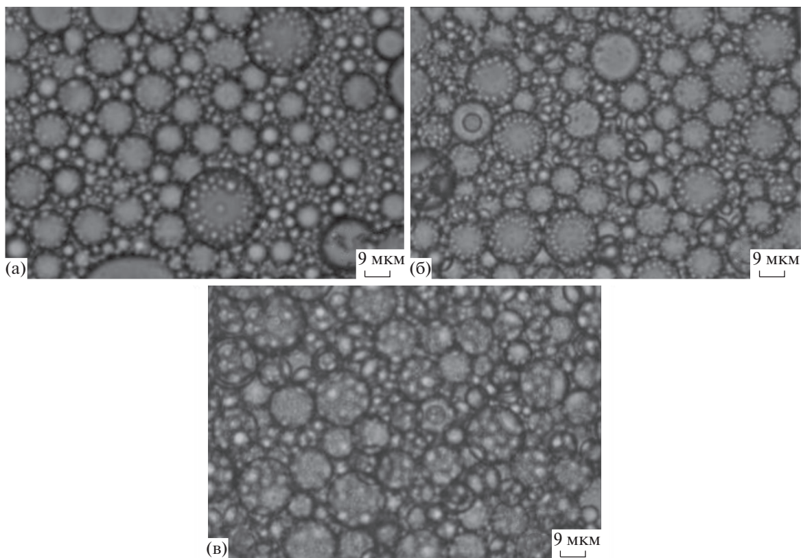
Рис. 6. Микрофотографии эмульсий с увеличением 40\times , содержащих наночастицы: (а) MWCNT; (б) \text{Fe}_2\text{O}_3 ; (в) \text{SiO}_2 .
