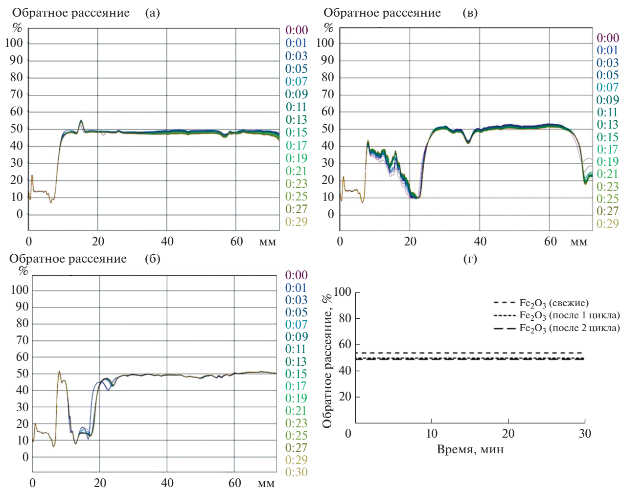
Рис. 9. Профили обратного рассеяния света эмульсией, содержащей \text{Fe}_2\text{O}_3 : (а) цикл 1; (б) цикл 2; (в) цикл 3; (г) средние профили обратного рассеяния света эмульсий, содержащих \text{Fe}_2\text{O}_3 .
