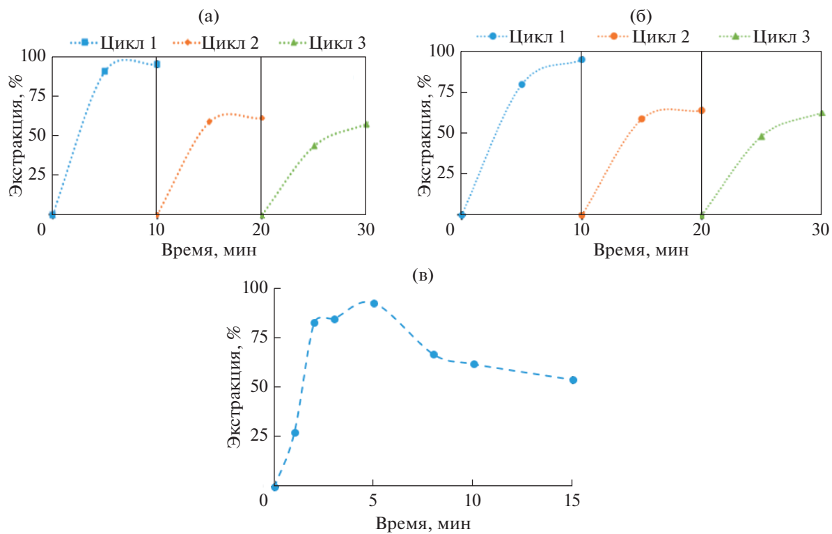
Рис. 7. Доля экстрагированного диклофенака при использовании эмульсионных наножидкостных мембран с наночастицами: (а) MWCNT; (б) \text{Fe}_2\text{O}_3 ; (в) \text{SiO}_2 .
