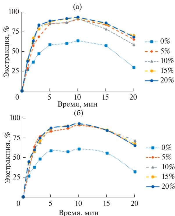
Рис. 12. Влияние наночастиц на степень извлечения диклофенака при использовании комбинации использованной и свежей эмульсий: (а) MWCNT; (б) Fe 2 O 3 .
