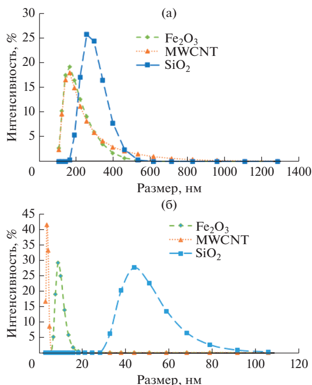
Рис. 5. Полученные методом динамического рассеяния света распределения по размерам (а) капель эмульсий в жидких мембранах; (б) наночастиц, использованных для стабилизации эмульсий.
