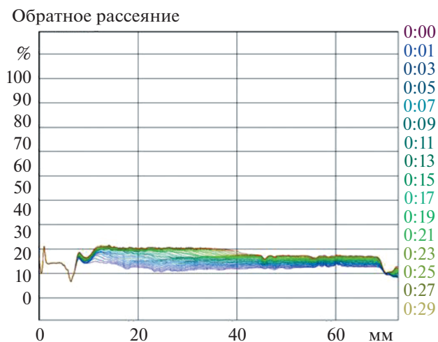
Рис. 10. Профили обратного рассеяния света эмульсией, содержащей SiO 2 .
