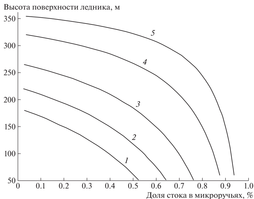
Рис. 4. Доля микропотоков в поверхностном стоке в зависимости от высоты поверхности ледника для разного запаса воды в коре таяния: 1 – 8 мм; 2 – 6 мм; 3 – 4 мм; 4 – 2 мм; 5 – 1 мм.
