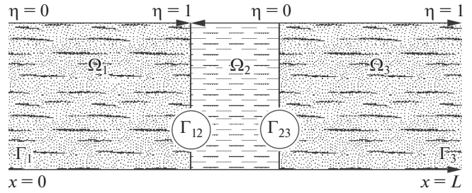
Рис. 2. Иллюстрация к математической модели. Fig. 2. Illustration to the mathematical model.
