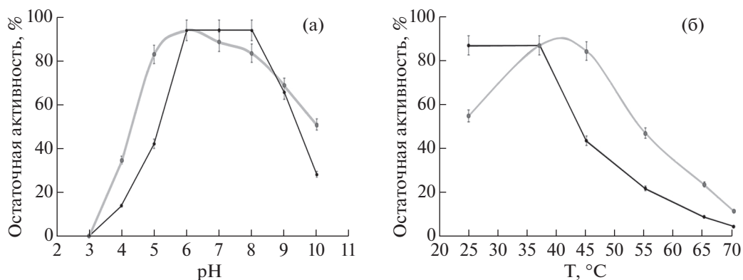
Рис. 2. Влияние pH (а) и температуры (б) на активность (черный график) и стабильность (серый график) препарата внеклеточных протеиназ микромицета Tolypocladium inflatum 62a.
