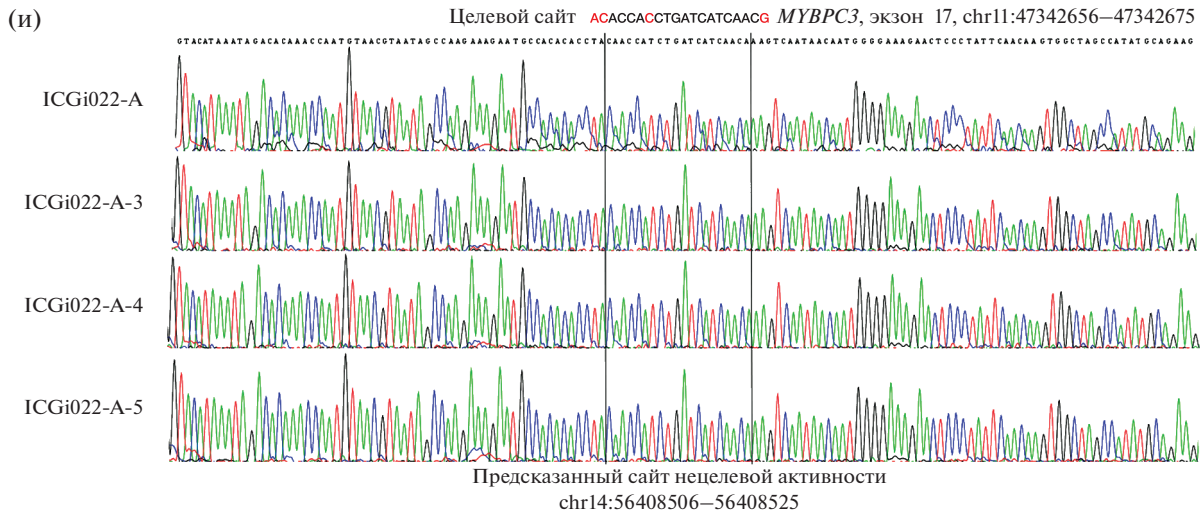
Рис. 1. Характеристика линий ИПСК ICGi022-A-3, ICGi022-A-4, ICGi022-A-5 с внесенной в ген MYBP3 мутацией р.Asn515del. (а) В трех линиях ИПСК, полученных в результате редактирования гена MYBP3 линии ИПСК ICGi022-A, выявлена гомозиготная мутация р.Asn515del. (б) Морфология линий ИПСК ICGi022-A-3, ICGi022-A-4 и ICGi022-A-5. Масштабная линейка – 200 мкм. (в) Экспрессия транскрипционных факторов OCT4 и NANOG и поверхностных антигенов TRA-1-60 и SSEA4 в полученных линиях ИПСК. Масштабная линейка – 100 мкм. (г) Анализ экспрессии генов OCT4 , NANOG , SOX2 методом ПЦР в реальном времени в линиях ИПСК ICGi022-A-3, ICGi022-A-4 и ICGi022-A-5. Линия эмбриональных стволовых клеток человека HUES9 была использована в качестве контроля. (д) Кариотип полученных линий ИПСК. (е) Подтверждение способности линий ИПСК ICGi022-A-3, ICGi022-A-4 и ICGi022-A-5 дифференцироваться в производные трех зародышевых листков. Масштабная линейка – 100 мкм. (ж) ПЦР-тест показал отсутствие в полученных линиях ИПСК эписомных векторов. (з) ПЦР-тест показал отсутствие контаминации линий ИПСК микоплазмами. (и) Отсутствие нецелевой активности системы CRISPR/Cas9 в линиях ИПСК ICGi022-A-3, ICGi022-A-4 и ICGi022-A-5 в предсказанном сайте нецелевой активности chr14:56408506–56408525.
