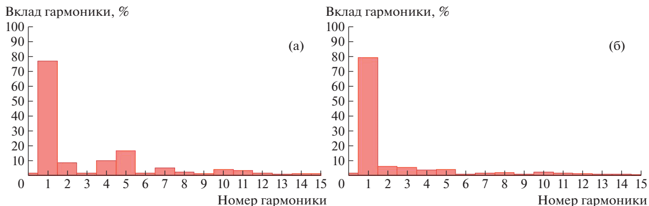
Рис. 6. Разложения тока фазы А по гармоникам: а – без дополнительных индуктивностей, б – с фильтрующими дросселями.
