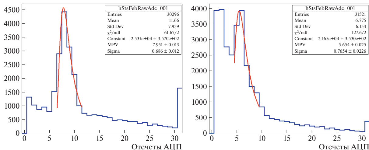
Рис. 7. Амплитуды сигналов от электронов с наиболее вероятной энергией 150 МэВ (слева) и 50 МэВ (справа). Собраный заряд составил 11.5 \pm 0.1 фКл для электронов с энергией 150 МэВ и 6.10 \pm 0.06 фКл для электронов с энергией 50 МэВ.
