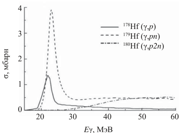
Рис. 4. Функции возбуждения реакций образования ^{177}\text{Lu} при облучении гафния тормозными фотонами [19, 29].
