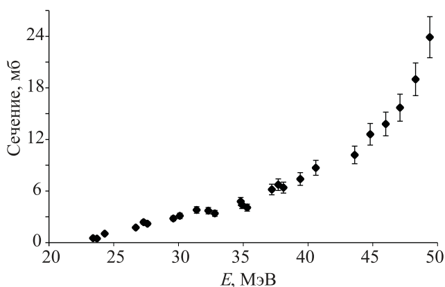
Рис. 5. Энергетическая зависимость сечений ядерных реакций ^{174}\text{Yb}(\alpha, x)^{177}\text{Lu} [22, 30]. 1
