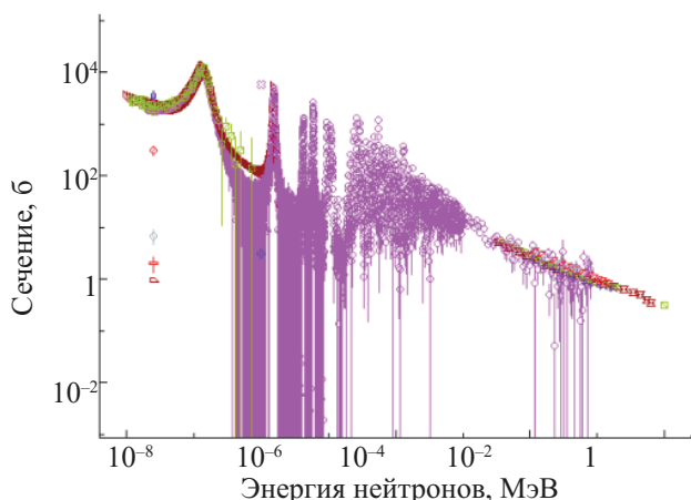
Рис. 1. Энергетическая зависимость сечений реакции ^{176}\text{Lu}(n,\gamma)^{177}\text{Lu} [19, 23, 24, 26, 27, 31].
