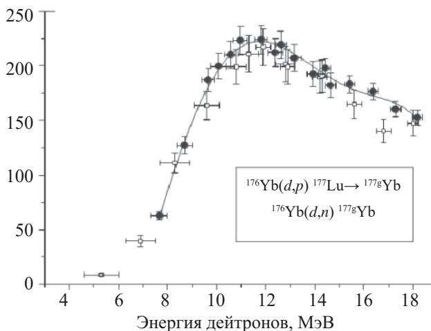
Рис. 3. Энергетическая зависимость сечений ядерных реакций получения ^{177}\text{Lu} ( ^{177}\text{Lu} ) на пучках дейтронов [19, 21, 25, 28].
