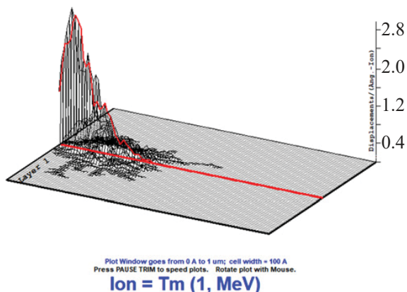
Рис. 7. Картина радиационных нарушений в металлической ^{176}\text{Yb} мишени в случае энергии ядер отдачи Tm, образовавшихся по каналам ( n,p ) или ( n,d ), равной 1 МэВ (диаметр зоны повреждений 1 мкм).
