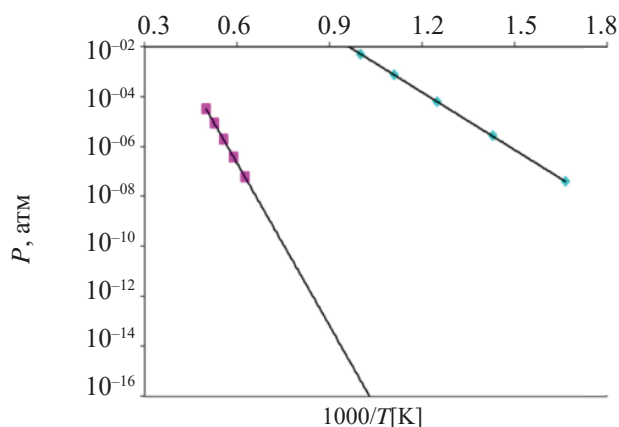
Рис. 6. Зависимость давления пара Yb и Lu от температуры. (Lu – красные точки, Yb – зеленые точки)
