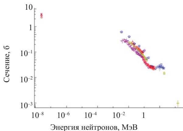
Рис. 2. Энергетическая зависимость сечений реакции ^{176}\text{Yb}(n,\gamma)^{177}\text{Yb} \rightarrow ^{177}\text{Lu} [19, 20].
