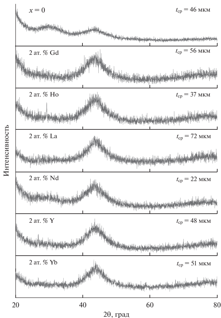
Рис. 3. Дифрактограммы сплавов (\text{Co}_{41}\text{Fe}_7\text{Cr}_{15}\text{Mo}_{14}\text{C}_{15}\text{B}_6)_{100-x}\text{R}_x ( \text{R} = \text{Gd}, \text{Ho}, \text{La}, \text{Nd}, \text{Y}, \text{Yb}; x = 0; 2 ), закаленных в форме лент.
