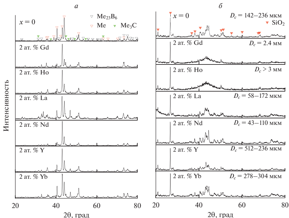
Рис. 1. Дифрактограммы закаленных сплавов (а) и стержней (б) (Co_{41}Fe_7Cr_{15}Mo_{14}C_{15}B_6)_{100-x}R_x (R = Gd, Ho, La, Nd, Y, Yb; x = 0; 2 ).
