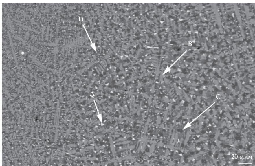
Рис. 2. СЭМ-изображение сплава состава \text{Co}_{41}\text{Fe}_7\text{Cr}_{15}\text{Mo}_{14}\text{C}_{15}\text{B}_6\text{Ho}_2 .
