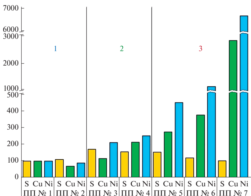
Рис. 2. Содержание элементов-загрязнителей (S, Cu, Ni) в лесной подстилке (горизонт O) на исследуемых ПП. Цифрами обозначены выделенные зоны загрязнения: 1 – фоновая (ПП № 1–2), 2 – буферная (ПП № 3–4), 3 – импактная (ПП № 5–7). По горизонтали – изучаемые элементы; по вертикали – изменения содержания элементов относительно контрольных (ПП № 1) значений (%).
