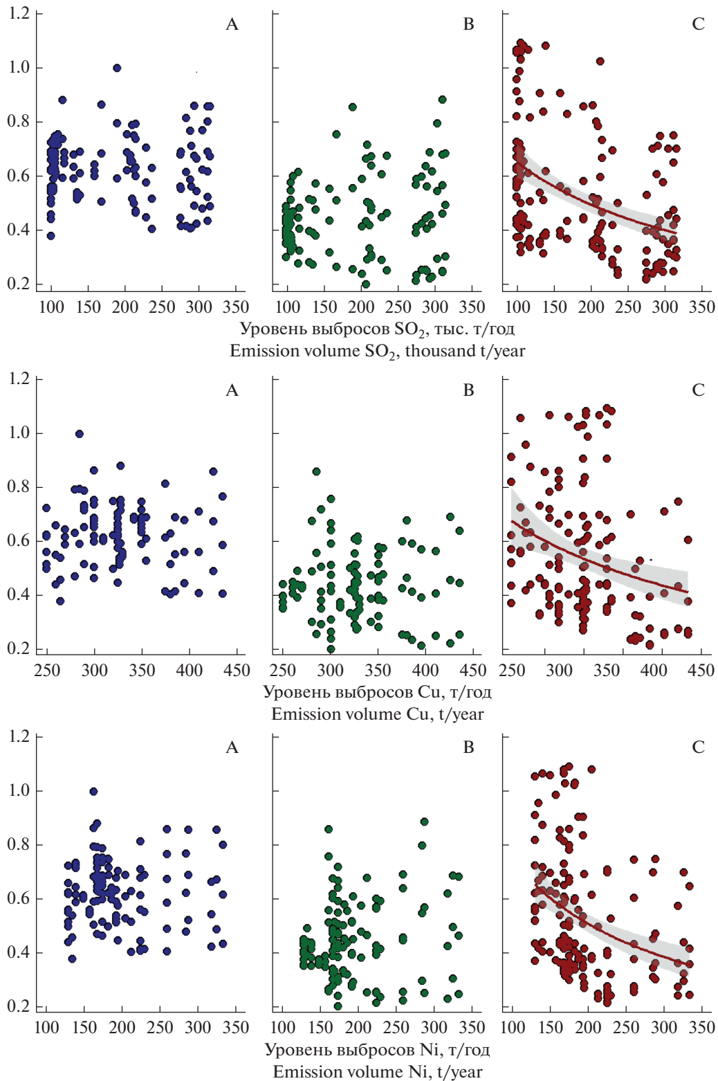
Рис. 5. Зависимость величины радиального прироста Pinus sylvestris от объемов выбросов основных загрязнителей ( \text{SO}_2 , Cu, Ni) в фоновой (A), буферной (B) и импактной (C) зонах.
