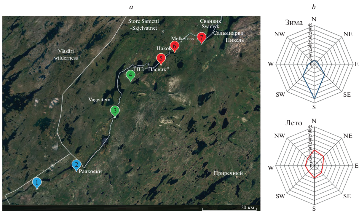
Рис. 1. a) Расположение постоянных ПП на разном удалении от источника аэротехногенного загрязнения (ГМК “Печенганикель”, пгт. Никель). Цветами обозначены зоны загрязнения: синий – фоновая (ПП № 1–2), зеленый – буферная (ПП № 3–4), красный – импактная (ПП № 5–7). b) Роза господствующих ветров в зимний и летний периоды в районе пгт. Никель.
