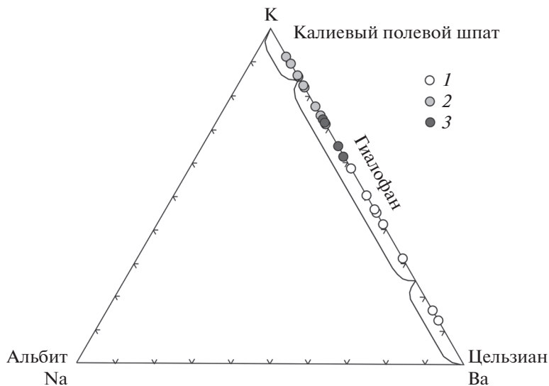
Рис. 6. Состав бариевого полевого шпата на диаграмме Na–K–Ba. Границы для калиевого полевого шпата, гялофана и цельзиана показаны в соответствии с работой (Essene et al., 2005). Бариевые полевые шпаты: 1 – из мельтейгита, 2 – ийолита, 3 – нефелинового сиенит-порфира.
