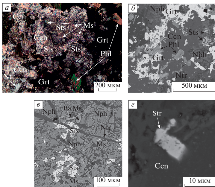
Рис. 3. Минералы Sr в породах массива.
