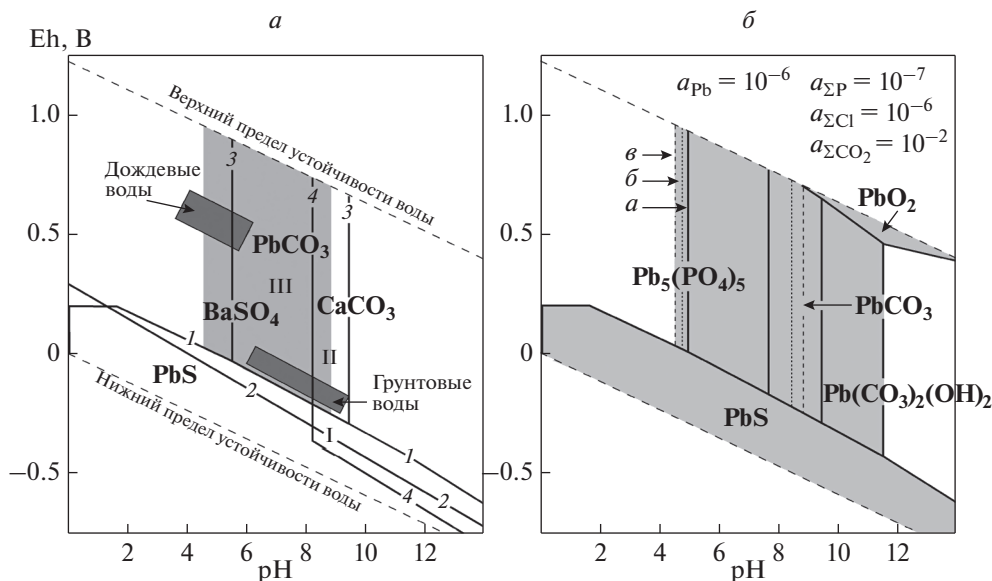
Рис. 6. Eh–pH диаграммы устойчивости минералов в воде при 25°C и 1 бар: a – для галенита, церуссита, барита, кальцита и пироморфита (Брусницын и др. 2022 b с дополнениями), б – для минералов свинца. На диаграмме a арабскими цифрами отмечены линии, ограничивающие поля устойчивости галенита (1), барита (2), церуссита (3) и кальцита (4). Римскими цифрами обозначены поля устойчивости минеральных ассоциаций первичных гидротермальных руд (I): кальцит + галенит + барит; слабо окисленных руд (II): кальцит + церуссит + барит; сильно окисленных руд (III): церуссит + барит. Светло-серым полем показана область устойчивости пироморфита (максимально большое поле на диаграмме б ), темно-серыми прямоугольниками показаны поля Eh–pH параметров для дождевых и грунтовых вод (Гаррелс, Крайст, 1968). Диаграмма построена для условий: активность растворенных свинца и бария – 10^{-6} , кальция – 10^{-4} , общей активности растворенных соединений серы и углерода – 10^{-2} . На диаграмме б серым цветом закрашены поля устойчивости твердых фаз, толстыми сплошными линиями ( a ) показаны границы устойчивости минералов при условиях показанных на рисунке, тонкими пунктирными – при условиях: ( б ) общей активности растворенных соединений фосфора – 10^{-7} , хлора – 10^{-4} , ( в ) общей активности растворенных соединений фосфора – 10^{-6} , хлора – 10^{-6} . Во всех случаях общая активность растворенных соединений серы – 10^{-2} . PbS – галенит, PbO 2 – платтнерит, PbCO 3 – церуссит, Pb 3 (CO 3 ) 2 (OH) 2 – гидроцеруссит, CaCO 3 – кальцит, BaSO 4 – барит, Pb 5 (PO 4 ) 3 Cl – пироморфит.
