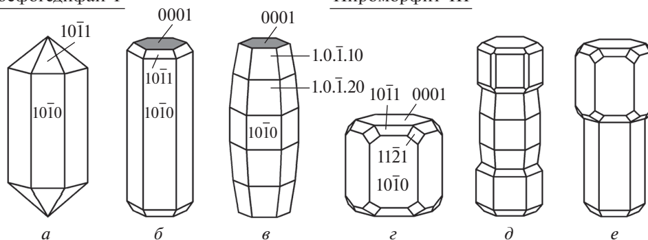
Рис. 1. Идеализированная морфология кристаллов фосфатов свинца. Габитус (и облик) кристаллов: a – дипирамидально-призматический, б – удлиненно-призматический, в – пинокоидально-пирамидальный (бочонковидный), г – коротко-столбчатый (пинокоидально-призматический), д и е – скипетровидные кристаллы с коротко-столбчатыми нарастаниями пироморфита на бочонковидные ( д ) и удлиненно-призматические ( е ) основания зонального Са-Pb фосфата. Серым цветом показаны грани пинакоида, имеющие неровную поверхность, образованную многочисленными бугорками роста.
