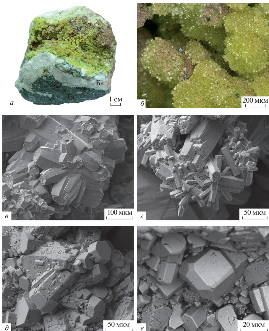
Рис. 2. Морфология выделения фосфатов свинца. Фотографии образцов: a и б – в отраженном свете, в – з – во вторичных электронах. a и б – сферолиты и друзы микроскопических кристаллов фосфатов свинца, обр. Уш-409: a – общий вид образца, б – деталь; в и з – незакономерные сростания (микродрузы) удлиненных кристаллов зонального Ca-Pb фосфата бочонковидного ( в ) и удлиненно-призматического облика ( з ), обр. Уш-409 (видно, что грани призмы и дипирамид ровные, а пинакоида – бугристые); д и е – септровидные кристаллы с коротко-столбчатыми нарастаниями пиломорфита на удлиненно-призматические основания зонального Ca-Pb фосфата, обр. Уш-403 (видно, что кристаллы пиломорфита обладают совершенными ровными гранями, тогда как грани Ca-Pb фосфата – “микроячейным”, блочным строением). Пористые скопления в центре кадра на рис. е – гётит. Га – галенит, Ба – барит.
