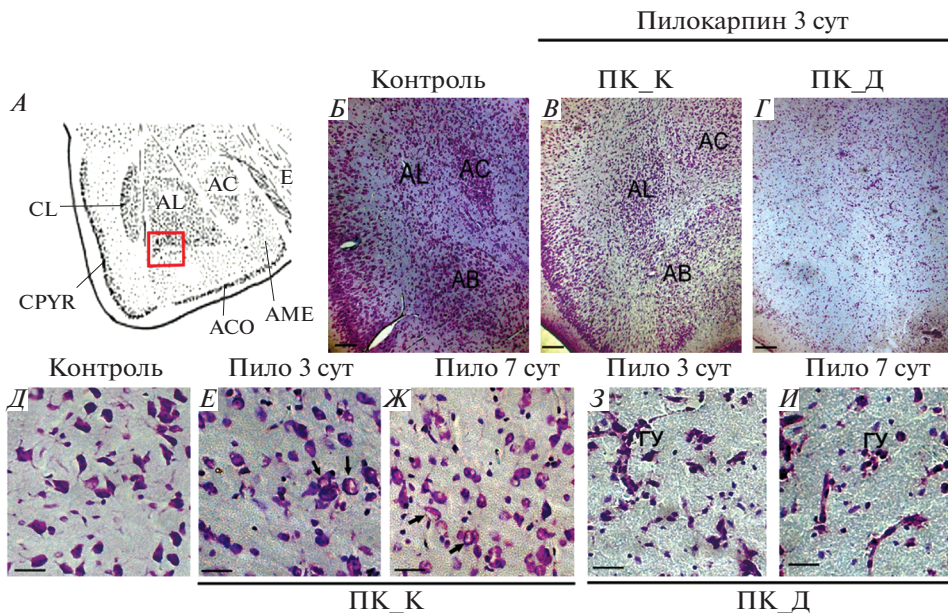
Рис. 2. Влияние литий-пилокарпиновых судорог на нервную ткань базолатеральной области миндалины крыс. Окрашивание по методу Ниссля. А – схема миндалины контрольных крыс. Обозначения: латеральное (AL), центральное (АС), базальное (AB) и медиальное (AME) ядра миндалины. Красной рамкой отмечена область базолатеральной миндалины на которой проводили морфометрический анализ. Б – участок ткани базолатеральной области миндалины контрольной крысы. Видно расположение ядер миндалины (обозначены так же, как на А ). В – участок ткани базолатеральной области миндалины крысы с краткосрочными судорогами (ПК_К), через 3-е сут после введения пилокарпина. Видно расположение ядер миндалины. Г – участок ткани базолатеральной области миндалины крысы с длительными судорогами (ПК_Д) через 3-е сут после введения пилокарпина. Массовая гибель нейронов не позволяет выявить границы ядер миндалины. Д – участок ткани базолатеральной области миндалины крысы при большем увеличении. Е–И – нейродегенеративные изменения в базолатеральной области миндалины крыс через 3-е ( Е, Г ) или 7 сут ( Ж, И ) после действия пилокарпина. У животных с краткосрочными судорогами ( Е, Ж ) отмечены нейродегенеративные изменения нейронов (отмечены стрелками) и незначительное повышение количества глиальных элементов. У животных с длительными судорогами ( З, И ) отмечено замещение нейронов глиальными элементами, в ткани заметны глиальные узелки (ГУ), свидетельствующие об активации глии при нейровоспалительном процессе. Масштаб: ( Д–И ) 20 мкм, ( Б–Г ) 100 мкм.
