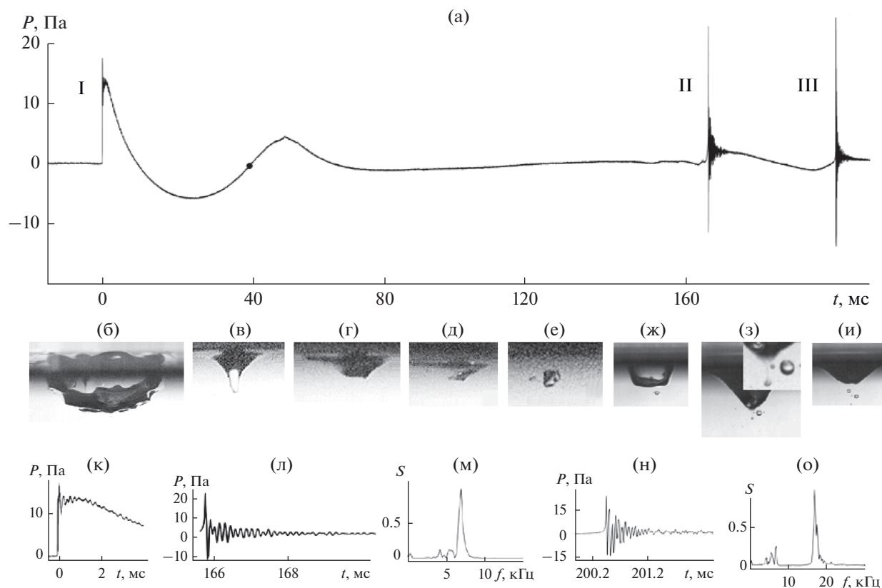
Рис. 5. (а) — Временная зависимость акустического давления с синхронными видеокдрами отрыва газовой полости. Деление 2 мм: (б) — каверна при t = 40.2 мс, (в)–(е) — формирующаяся и отрывающаяся газова́я полость при t = 163.7 , 165.2, 165.5, 166.2 мс; (ж)–(и): новая каверна (186.2 мс), формирование (200.5 мс, увеличенный фрагмент на (з)) и отрыв донной газовой полости (203.5 мс); (к) и (л) — растянутые ударный импульс и пакет II, (м) — спектр пакета II, (н) и (о) — растянутый пакет III и его спектр. D = 0.5 см, U = 3.2 м/с, We = 701 , Re = 16000 , Fr = 209 , Oh = 0.0017 , Bo = 3.4 .
