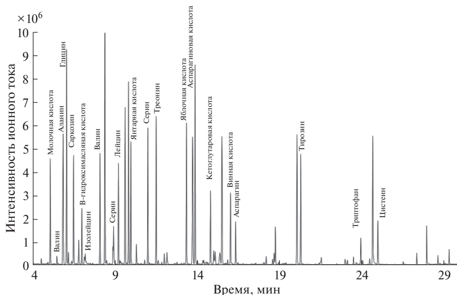
Рис. 5. Хроматограмма раствора стандартов аминокислот и низкомолекулярных органических кислот в форме силильных производных, полученная методом ГХ-МС. Условия ГХ-МС: газовый хромато-масс-спектрометр Shimadzu GCMS-QP2010 Ultra, хроматографическая колонка HP-5 (30 м × 0.320 мм × 0.25 мкм, Agilent); газ-носитель — гелий, скорость потока — 1.2 мл/мин; температурный градиент: 50–300°C со скоростью 10°C/мин; температура испарителя — 250°C; объем пробы — 1 мкл; масс-спектрометр в режиме сканирования ионов (EI 70 эВ, температура ионного источника 250°C, диапазон масс m/z 50–450 Да).
