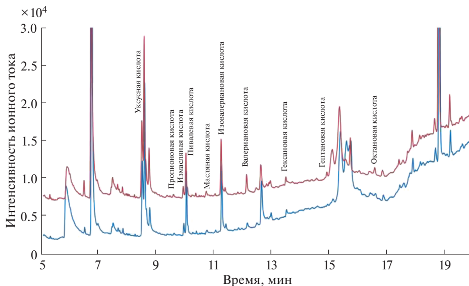
Рис. 7. Сравнение хроматографических профилей по выделенному ионному току органических кислот в сыворотке крови пациенток с диагнозами миома матки (синий цвет) и эндометриоз (красный цвет), полученных методом ГХ-МС без дериватизации.
