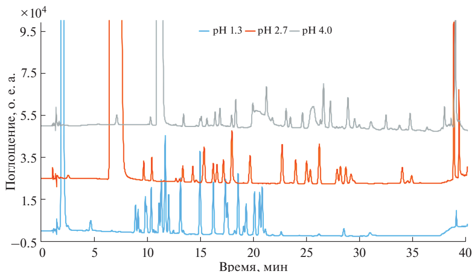
Рис. 1. Хроматограммы смесей стандартов аминокислот в виде производных с дансилхлоридом, полученные методом ОФ ВЭЖХ при различных значениях pH подвижной фазы. Условия ОФ ВЭЖХ-анализа: колонка Luna C18(2) 150 мм × 2.1 мм × 5 мкм; температура колонки +30°C, скорость потока подвижной фазы 0.3 мл/мин; 280 нм. Градиентный режим элюирования (см. табл. 1); подвижная фаза: хроматограмма серого цвета : фаза А – 50 мМ ацетатный буферный раствор с pH 4.0, фаза Б – ацетонитрил; хроматограмма оранжевого цвета : фаза А – 0.1%-ный водный раствор HCOOH (pH 2.7), фаза Б – 0.1%-ный раствор HCOOH в ацетонитриле; хроматограмма синего цвета : фаза А – 0.05%-ный водный раствор трифторуксусной кислоты (pH 1.3), фаза Б – ацетонитрил.
