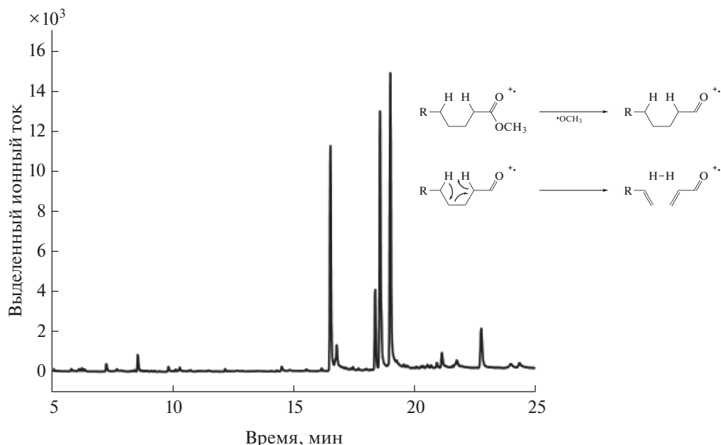
Рис. 4. Характеристический профиль жирных кислот в образце сыворотки крови с миомой матки. GCMS-QP2010 SE с квадрупольным масс-селективным детектором с электронной ионизацией пробы. Хроматографическая колонка WAXplus (OPTIMA 30 м × 0.25 мм × 0.25 мкм). Режим SIM: m/z 55. Режим программирования температуры.
