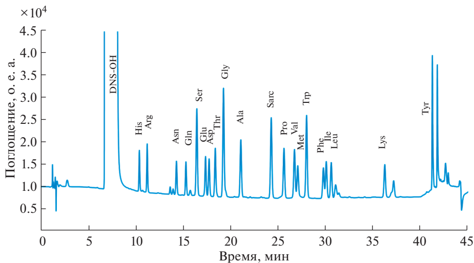
Рис. 2. Хроматограмма смеси стандартов аминокислот в форме дансильных производных. Условия: колонка Luna C18(2) 150 мм × 2.1 мм × 5 мкм; температура колонки: +30°C; 280 нм; скорость потока подвижной фазы 0.3 мл/мин; градиентный режим: фаза А – H 2 O, 0.1% HCOOH (pH 2.7), фаза Б – ацетонитрил, 0.1% HCOOH.
