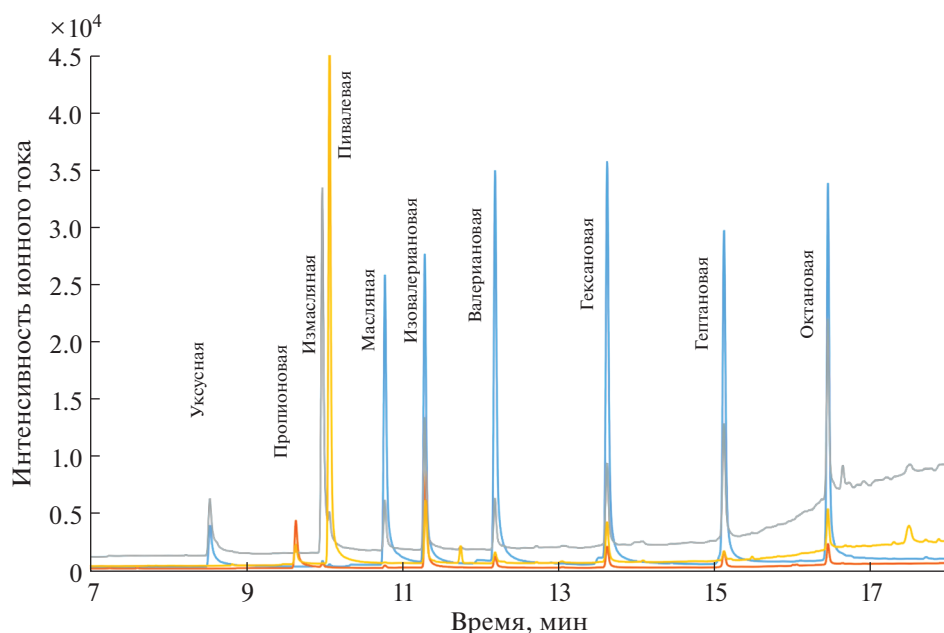
Рис. 6. Хромограмма по ионному току выделенных масс стандартов низкомолекулярных жирных органических кислот C2–C8 (5 мкг/мл), полученная методом ГХ-МС на капиллярной колонке ZB FFAP (Phenomenex). Условия: газовый хромато-масс-спектрометр Shimadzu GCMS-QP2010 Ultra, хроматографическая колонка Zebron ZB FFAP 50 м × 0.32 мм × 0.50 мкм (Phenomenex); газ-носитель — гелий, скорость потока — 1.5 мл/мин; температурный градиент: 70–200°C со скоростью 10°C/мин; температура испарителя — 200°C; объем пробы — 1 мкл; масс-спектрометр в режиме сканирования ионов (EI 70 эВ, температура ионного источника 250°C, диапазон масс m/z 50–450 Да).
