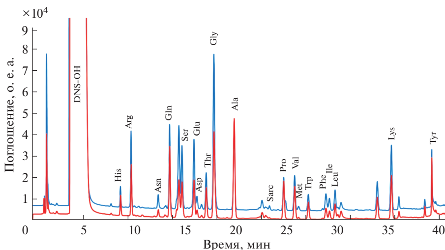
Рис. 3. Хроматограммы дансильных производных аминокислот в сыворотке крови больных с диагнозами эндометриоз (красный цвет) и миома матки (синий цвет) (ОФ ВЭЖХ). Условия: колонка Luna C18(2) 150 мм × 2.1 мм × 5 мкм; температура колонки +30°C; 280 нм; скорость потока подвижной фазы 0.3 мл/мин; градиентный режим элюирования: фаза А – 0.1%-ный водный раствор HCOOH (pH 2.7), фаза Б – 0.1%-ный раствор HCOOH в ацетонитриле.
