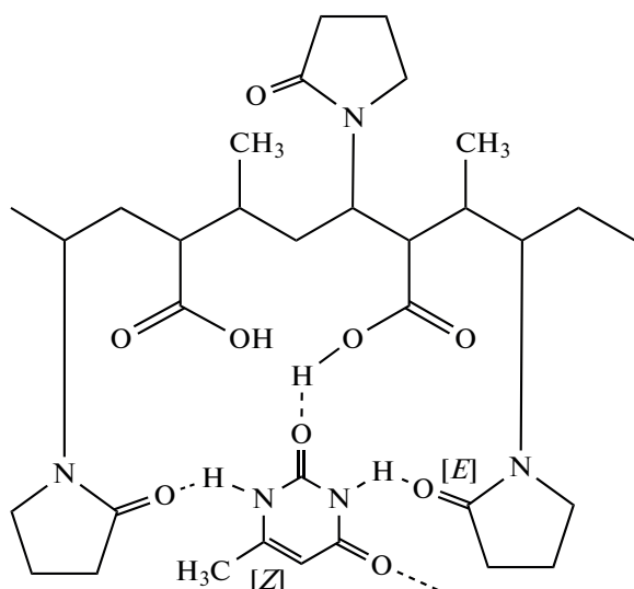
Схема 5. Структурная формула конъюгата и полимера-носителя с “Метилурацилом”.
