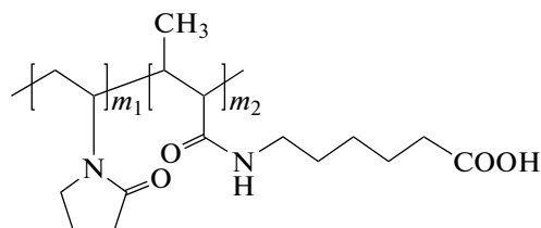
Схема 2. Структурная формула сополимера N-ВП–6-КАКК.
