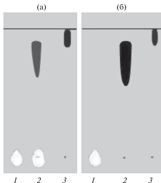
Рис. 3. Хроматограммы сополимера винилпирролидон (ВП)–6-кротоноиламинокапроновой кислоты (6-КАКК) до (а) и после очистки (б). 1 – 6-КАКК, 2 – сополимер ВП–6-КАКК, 3 – поливинилпирролидон 40000 Да.
