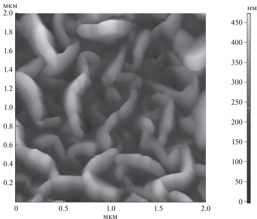
Рис. 2. АСМ-изображение поверхности керамики, покрытой фторопластом методом электронно-лучевого диспергирования в вакууме.
