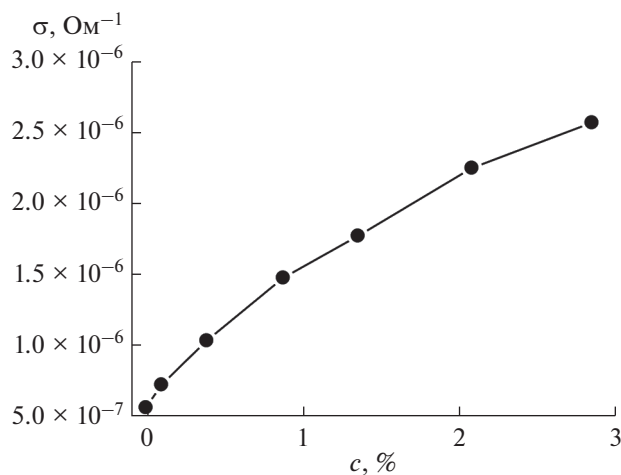
Рис. 4. Зависимость проводимости сенсора ( \sigma ) от концентрации метана ( c ) в барботирующем через воду очищенном воздухе.
