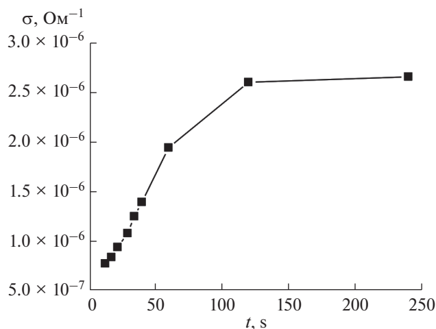
Рис. 3. Зависимость электропроводности сенсора ( \sigma ) от времени ( t ) пребывания газа-носителя внутри трубчатой мембраны.
