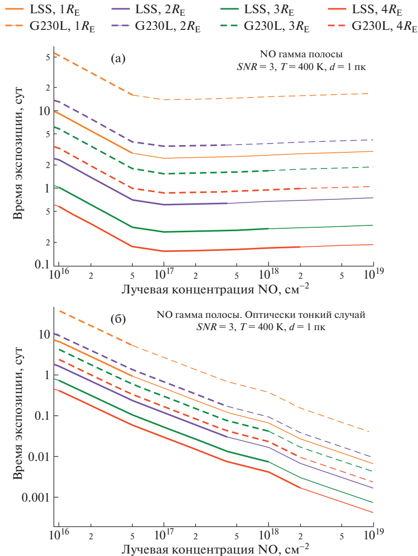
Рис. 3. Значения времени экспозиции для наблюдения эмиссии в системе \gamma -полосы NO на разных модельных планетах, находящихся на расстоянии 1 пк в следующих случаях: а) оптически толстый случай, SNR = 3 , б) оптически тонкий случай, SNR = 3 . Оранжевые линии соответствуют экзo-Землям с 1R_E , фиолетовые линии – супер-Землям с 2R_E , зеленые линии – суб-Нептунам с 3R_E и красные линии – суб-Нептунам с 4R_E . Пунктирные линии соответствуют вычислениям с параметрами COS G230L и сплошные линии – вычислениям с параметрами LSS.
