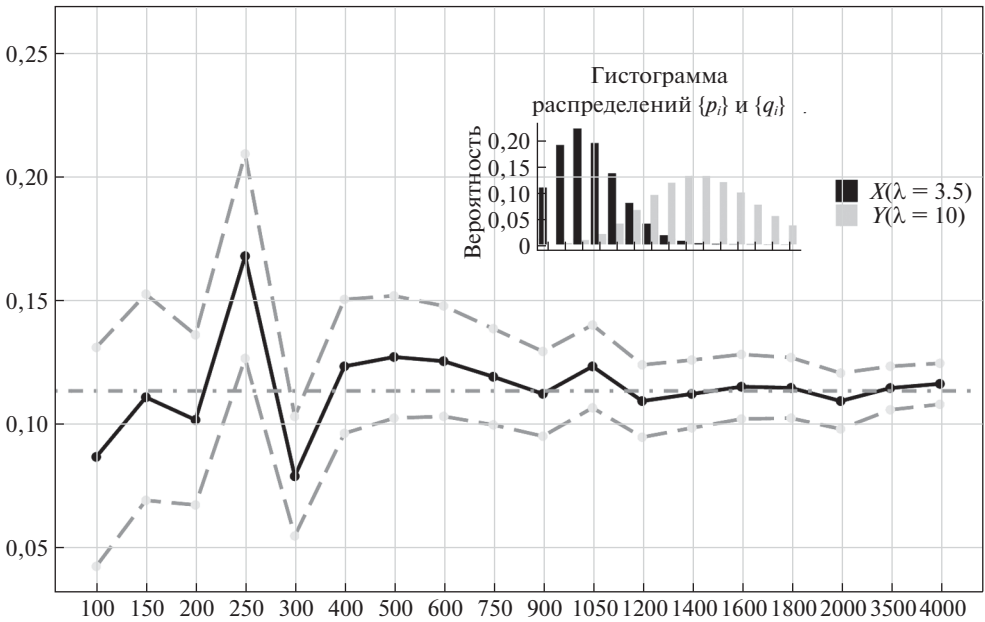
Рис. 3. Доверительные границы для меры сходства Ружички и значения частотного индекса Ружички для выборок X и Y из усеченных распределений Пуассона с параметрами a - (5, 10) и b - (3,5, 10) в зависимости от n, m = n .
