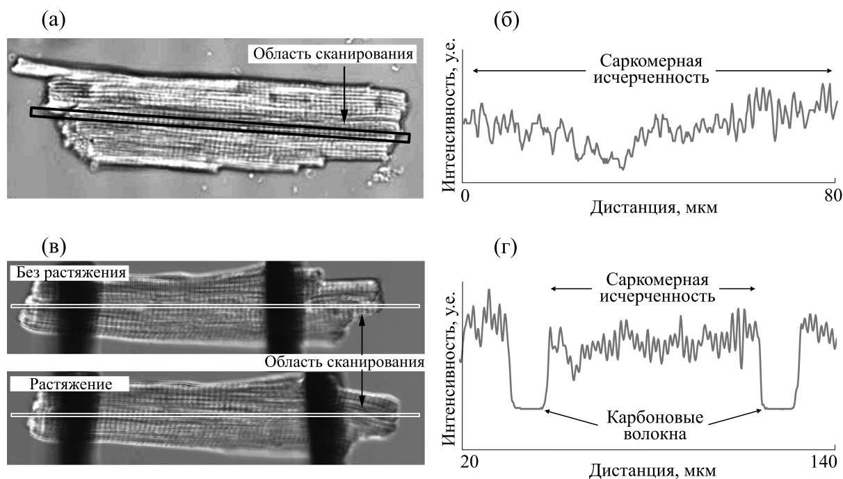
Рис. 1. Регистрация профиля саркомерной истерченности в изолированном кардиомиоците: (а) — изображение кардиомиоцита в ненагруженном режиме сокращения; (б) — пример профиля интенсивности изображения кардиомиоцита при сокращении в ненагруженном режиме; (в) — изображение кардиомиоцита в нерастянутом и растянутом состоянии при использовании карбоновых волокон; (г) — пример профиля интенсивности изображения кардиомиоцита при сокращении в нагруженном режиме с использованием карбоновых волокон, области с минимальной интенсивностью соответствуют положениям волокон. На панелях (а) и (в) показана область, для которой строится профиль интенсивности изображения кардиомиоцита. Данные на панелях (в) и (г) адаптированы и модифицированы из работы [13].
