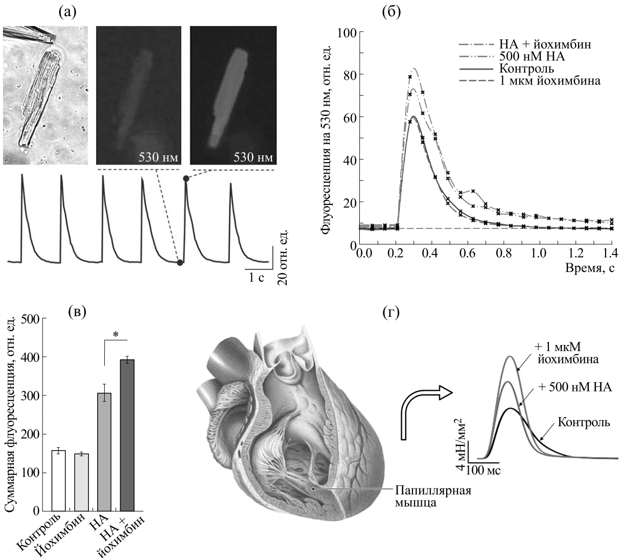
Рис. 4. Активация \alpha_2 -AR уменьшает внутриклеточную \text{Ca}^{2+} -нагрузку. (а) – Одиночный кардиомиоцит, нагруженный \text{Ca}^{2+} -красителем Fluo-4AM, в проходящем свете и флуоресцирующий на длине волны 530 нм в ответ на стимуляцию с частотой 1 Гц через приближенный стеклянный электрод. (б) – Сравнительные одиночные \text{Ca}^{2+} -переходы, измеренные последовательно в контроле, в присутствии антагониста \alpha_2 -AR йохимбина и в присутствии норадреналина, который вызывал значительное увеличение внутриклеточного \text{Ca}^{2+} . Блокирование йохимбином активированных норадреналином \alpha_2 -AR вызывало дополнительную внутриклеточную \text{Ca}^{2+} -нагрузку. (в) – Статистика, соответствующая панели (б). (г) – Записи изометрического сокращения изолированной папиллярной мышцы при стимуляции с частотой 1 Гц. Согласно увеличению внутриклеточного \text{Ca}^{2+} в присутствии норадреналина и йохимбина, блокирование \alpha_2 -AR усиливало норадреналин-зависимую сократительную нагрузку папиллярной мышцы (адаптировано из работы [63]).
