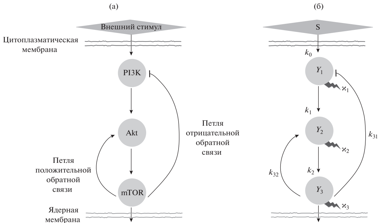
Рис. 2. Схематическая диаграмма каскада PI3K–Akt–mTOR, содержащая названия участвующих белков и обозначения петель обратных связей (а) и введенные символичные обозначения (б).
