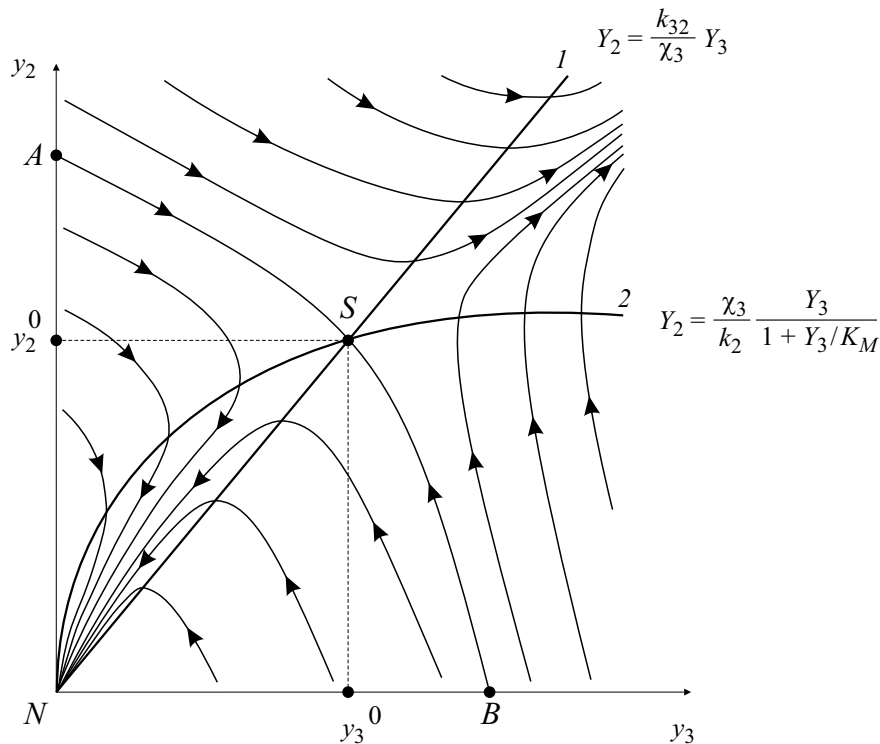
Рис. 3. Фазовый портрет динамической системы (4)–(5). Линии 1 и 2 – нуль-изоклины. Особые точки: N – устойчивый узел, S – седло. Сепаратриса ASB разделяет два динамических режима в фазовом пространстве системы: релаксация к устойчивому исходному состоянию и передача сигнала с нарастанием динамических переменных.
