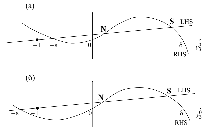
Рис. 4. Графическое представление решений уравнения (17). Рассмотрены два варианта расположения точек пересечения: а) \varepsilon < 1 и б) \varepsilon > 1 . В обоих случаях один из корней нефизичен (отрицательное значение концентрации). Далее при рассмотрении ограничение на параметр \varepsilon > 0 .
