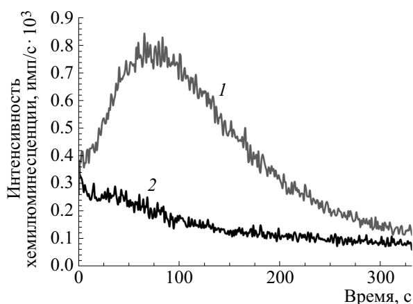
Рис. 6. Суммарная интенсивность хемилюминесценции в диапазоне длин волн 300–650 нм смеси начального состава: 10 мкМ цитохрома c , 300 мкМ ТОКЛ, 215 мкМ \text{H}_2\text{O}_2 без добавления производного кумарина (кривая 1) и в присутствии 25 мкМ С-334 (кривая 2).
