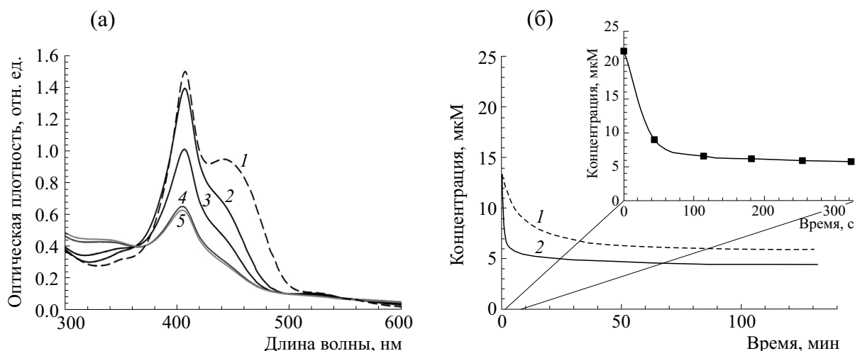
Рис. 5. Пероксидазная реакция в системе начального состава: 10 мкМ цитохрома c , 300 мкМ ТОКЛ, 25 мкМ С-525, 215 мкМ \text{H}_2\text{O}_2 . (а) – Серия спектров поглощения смеси: 1 – спектр поглощения смеси без \text{H}_2\text{O}_2 , 2 – спектр поглощения через 15 с после начала реакции, 3 – через 5 мин, 4 – через 59 мин, 5 – через 120 мин. (б) – Уменьшение концентрации цитохрома c (кривая 1) и С-525 (кривая 2) в процессе реакции, на врезке – уменьшение концентрации С-525 в первые минуты реакции.
