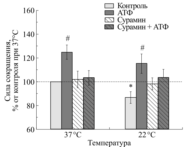
Рис. 2. Влияние температуры на силу сокращений m. Diafragma крысы, вызванных карбахолином, в отсутствие и в присутствии АТФ (100 мкМ) и сурамина (100 мкМ). Результаты представлены в виде M \pm m в % от исходных величин, принятых за 100%; n = 12 ; * – p < 0.05 от эффекта при 37°C, # – p < 0.05 от контроля.
