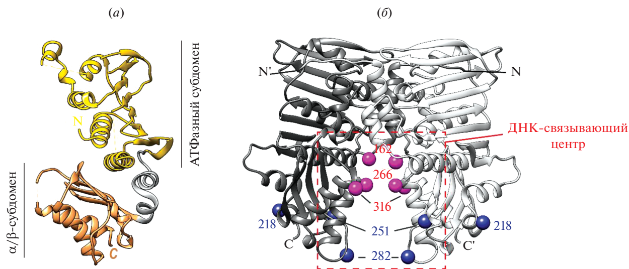
Рис. 7. Строение N-концевого домена MutL из E. coli . (a) Кристаллическая структура мономера MutL-NTD (PDB: 1BKN). Желтым цветом отмечен АТФазный субдомен, коричневым — \alpha/\beta -субдомен. (b) Кристаллическая структура димера MutL-NTD в комплексе с AMP-PNP (PDB: 1B63). Розовыми сферами обозначены остатки Arg, необходимые для связывания ДНК согласно [19], синими — остатки, сближенные с ДНК в процессе функционирования белка согласно [107]. Красной пунктирной рамкой указана предполагаемая ДНК-связывающая область MutL.
