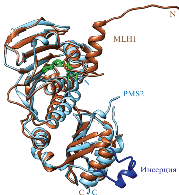
Рис. 5. Совмещение кристаллических структур АТФазных доменов белков MLH1 и PMS2 в комплексе с АТР и АТР \gamma S соответственно (PDB: 3NA3, 1H7U). Синим цветом обозначена инсерция пептида в белке PMS2, зеленым — нуклеотидные кофакторы АТР и АТР \gamma S.
