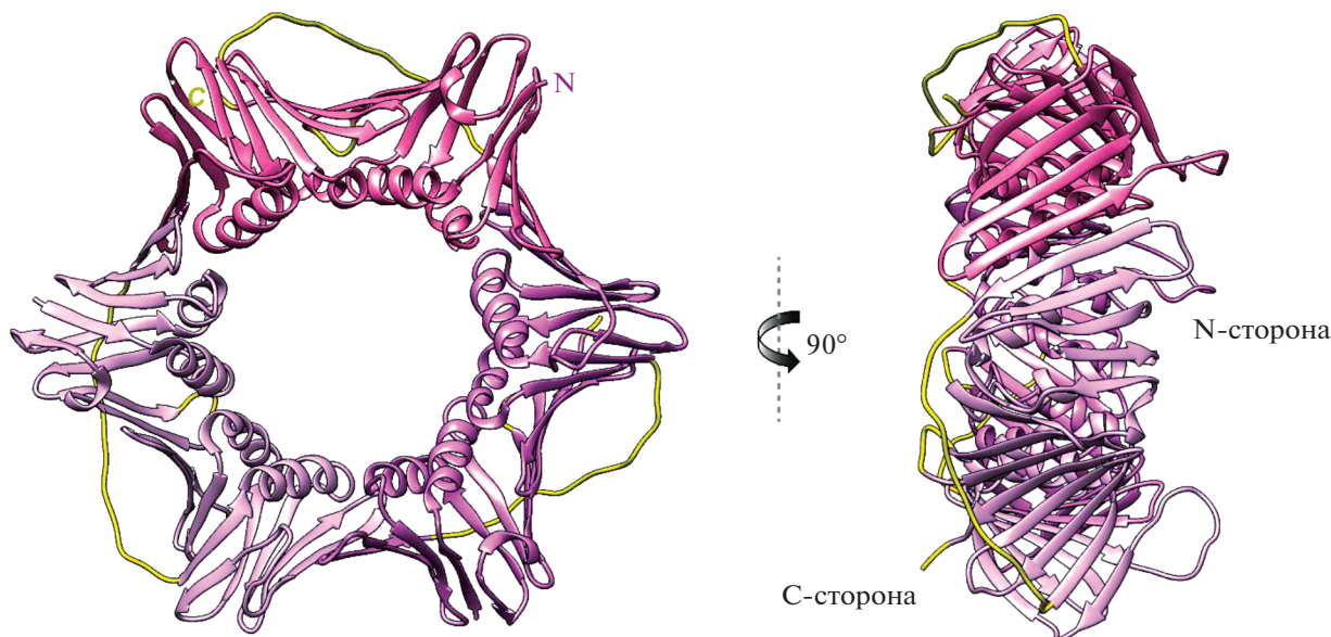
Рис. 1. Кристаллическая структура PCNA человека (PDB: 1VYM) в двух проекциях. Желтым обозначены гидрофобные участки С-стороны белка, участвующие во взаимодействии с белковыми партнерами.
