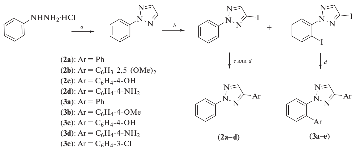
Схема 2. Синтез соединений ( 2 ) и ( 3 ). Реагенты и условия реакций: a – NaOH, (CHO) 2 , Cu(OTf) 2 , t ; b – 1. ZnCl 2 ·TMEDA, LiTMP, THF, комн. темп., 2 ч; 2. I 2 , комн. темп., 2 ч; c – ArB(OH) 2 , Pd(dba) 2 , PPh 3 , CsF, диоксан, кипячение; d – ArB(OH) 2 , PdCl 2 , PPh 3 , Na 2 CO 3 , H 2 O, EtOH, DME, кипячение.
