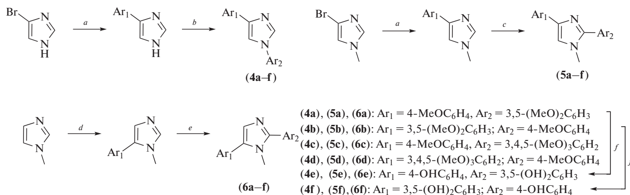
Схема 3. Синтез соединений ( 4–6 ). Реагенты и условия реакций: a – Ar 1 B(OH) 2 , PdCl 2 (dppf), VnEt 3 NCl, CsF, толуол, H 2 O, 110°C; b – Ar 2 Br, (CuOTf) 2 ·PhMe, 1,10-фенантролин, dba, Cs 2 CO 3 , ксилол, 110°C; c – Ar 2 Br, Pd(OAc) 2 , CuI, DMA, 160°C; d – Ar 1 Br, Pd(OAc) 2 , n -Bu 4 NOAc, DMA, 110°C; e – Ar 2 Br, CuI, 110°C; f – BBr 3 , CH 2 Cl 2 , –60°C, MeOH.
