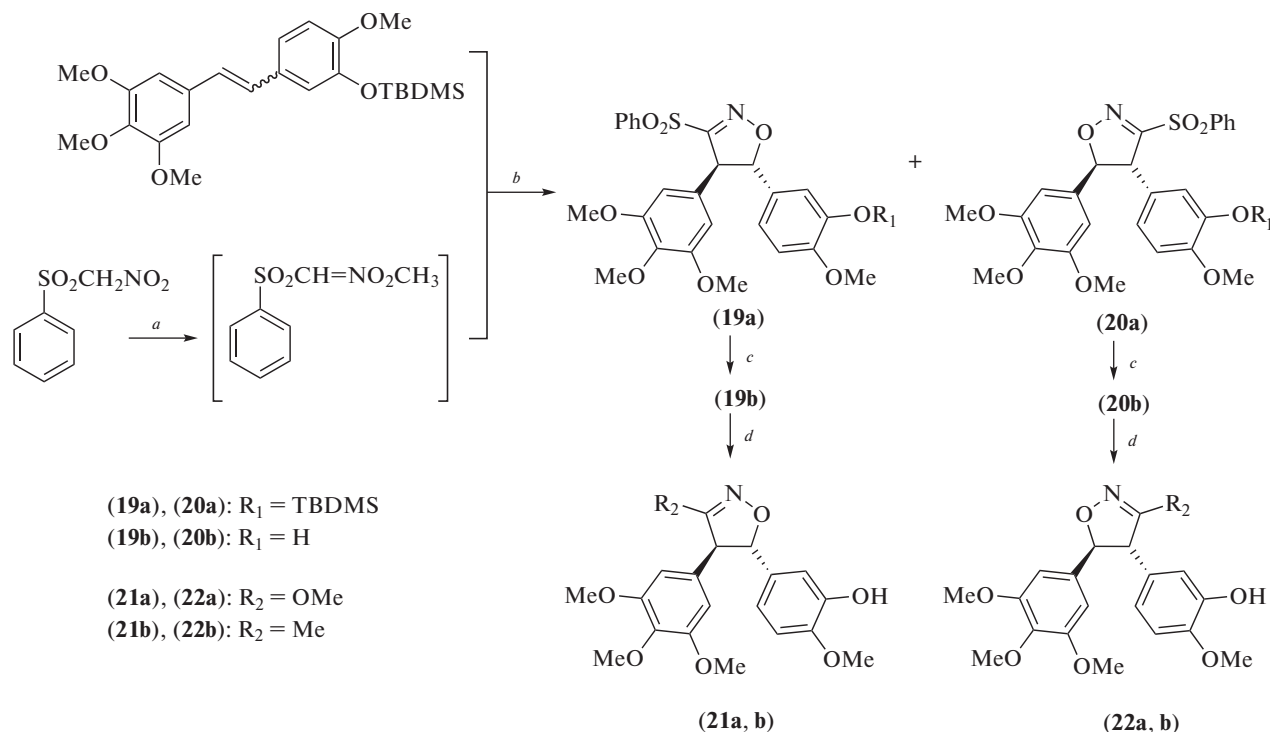
Схема 11. Синтез соединений (19–22). Реагенты и условия реакций: a – diazometan, Et 2 O; b – CH 2 Cl 2 , n -TsOH, кипячение; c – TBAF, CH 2 Cl 2 ; d – Na, CH 3 OH или MeLi, THF.
