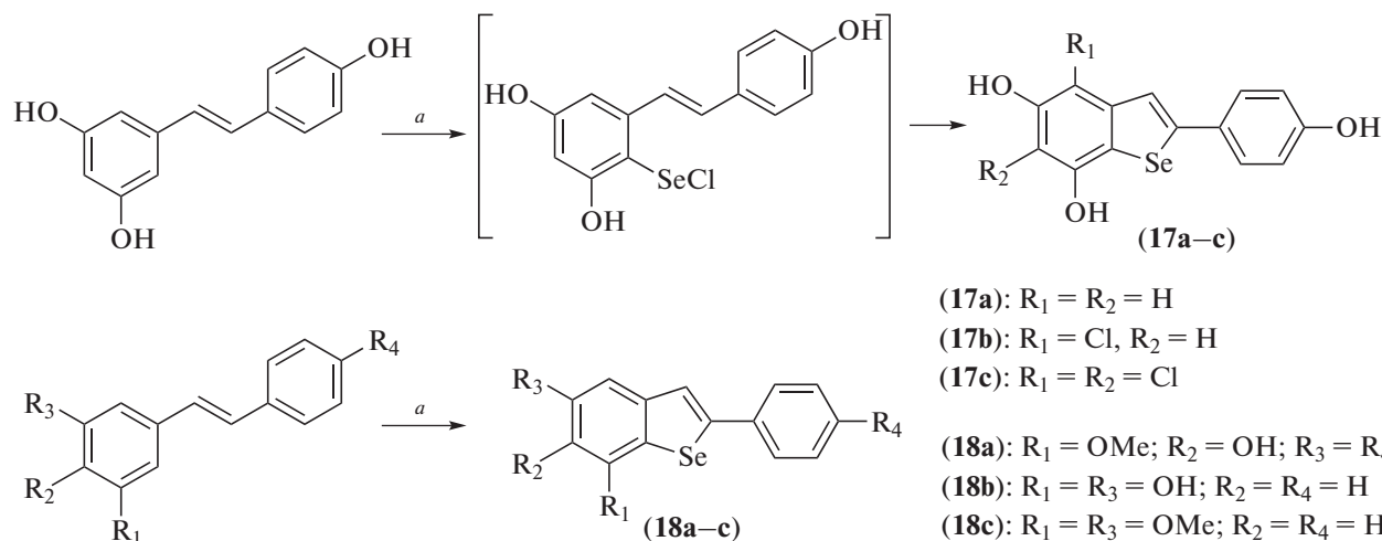
Схема 10. Синтез соединений (17) и (18). Реагенты и условия реакций: a – 1. Se, SO_2Cl_2 , THF; 2. DMF, комн. темп.
