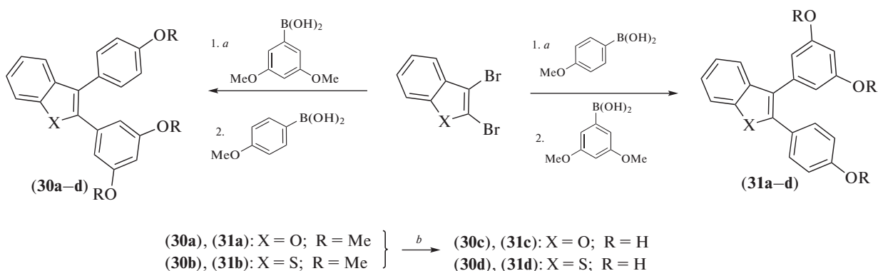
Схема 17. Синтез соединений (30) и (31). Реагенты и условия реакций: a – \text{Pd}(\text{PPh}_3)_4 , 2 М \text{Na}_2\text{CO}_3 , толуол/ \text{EtOH} 3 : 1, кипячение, 6 ч; b – 1 М \text{BBr}_3 , \text{CH}_2\text{Cl}_2 , комн. темп., 20 ч.
