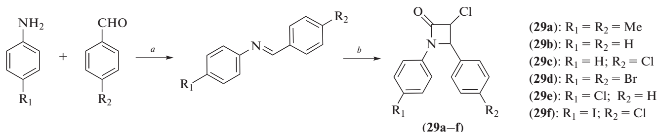
Схема 16. Синтез соединений (29). Реагенты и условия реакций: a – толуол; b – 2-хлорацетилхлорид, ТЕА, \text{CH}_2\text{Cl}_2 , -78^\circ\text{C} .
