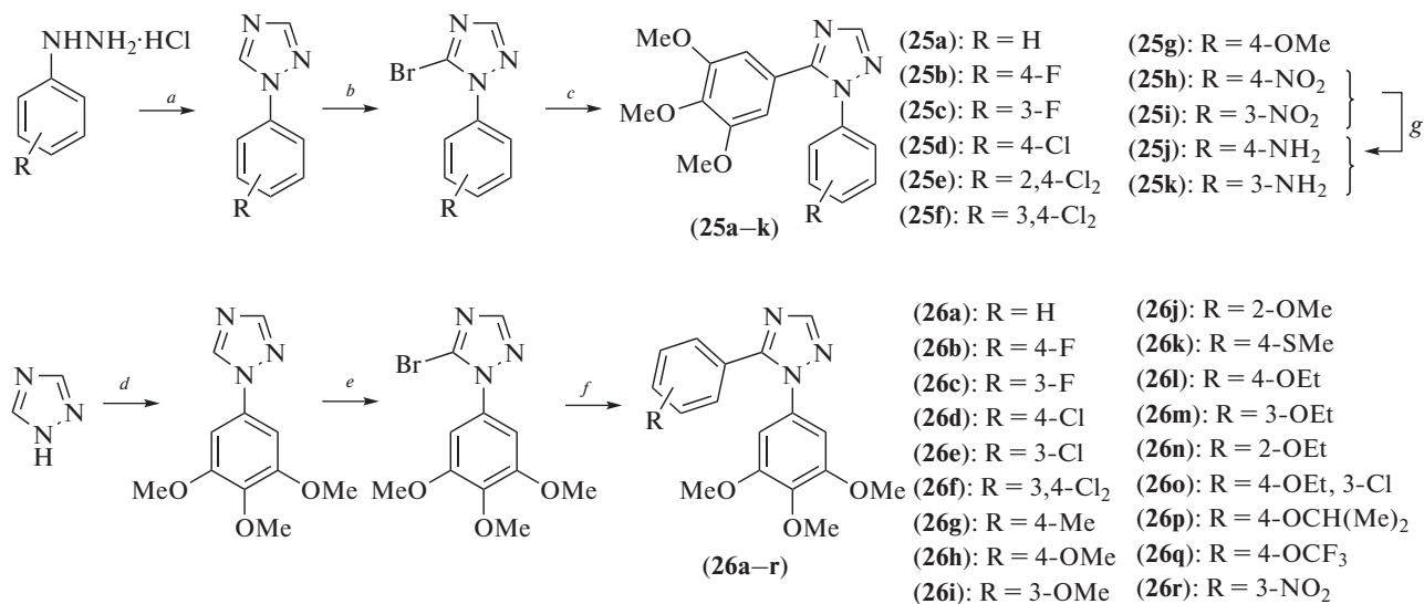
Схема 13. Синтез соединений ( 25 ) и ( 26 ). Реагенты и условия реакций: a – HCONH 2 , 120°C, 18 ч; b, e – NBS, бензоилпероксид (кат.), CCl 4 , кипячение; c, f – Pd(PPh 3 ) 4 , K 2 CO 3 , PhMe, кипячение, 18 ч; d – 1-бром-3,4,5-триметоксибензол, CsCO 3 , CuI, DMF, 120°C, 18 ч; g – H 2 , 10% Pd/C, DMF.
