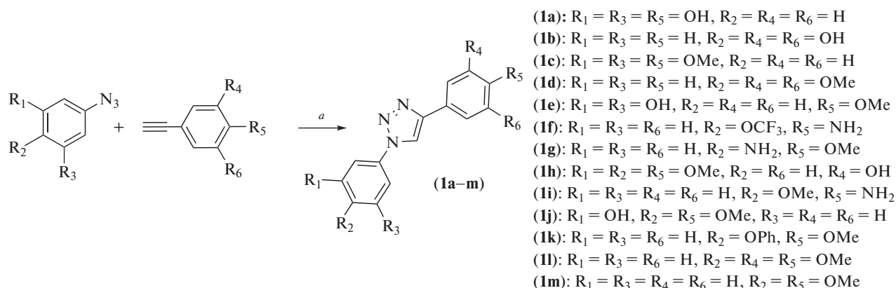
Схема 1. Синтез соединений ( 1 ). Реагенты и условия реакций: a – CuSO 4 , аскорбат натрия, H 2 O, t -BuOH.
