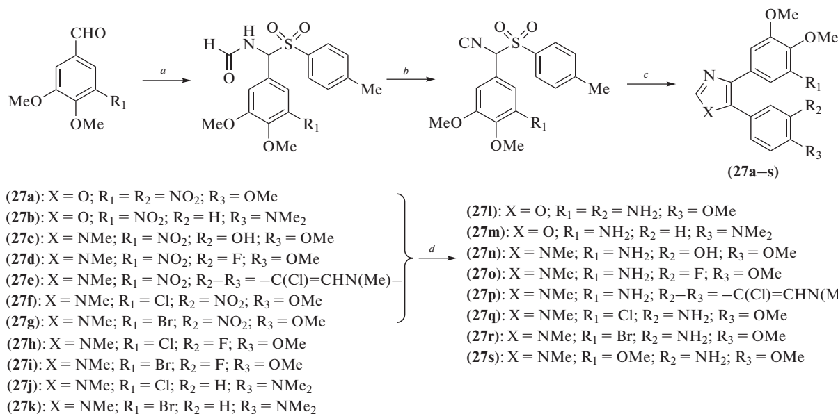
Схема 14. Синтез соединений (27). Реагенты и условия реакций: a – HCONH 2 , CSA, n -толуолсульфиновая кислота, 16 ч, 60°C; b – POCl 3 , Et 3 N, DME, 3 ч, –5°C; c – AgCHO, K 2 CO 3 , DME/MeOH, 2 ч, кипячение (для X = O) или AgCHO, MeNH 2 (33% в EtOH), AcOH, EtOH, 2 ч, кипячение (для X = NMe); d – HCO 2 NH 4 , Pd/C (5%), MeOH, 2 ч, кипячение (для соединений (27a–d)) или Zn, HCl, THF, 10 мин, комн. темп. (для соединений (27e–g)).
