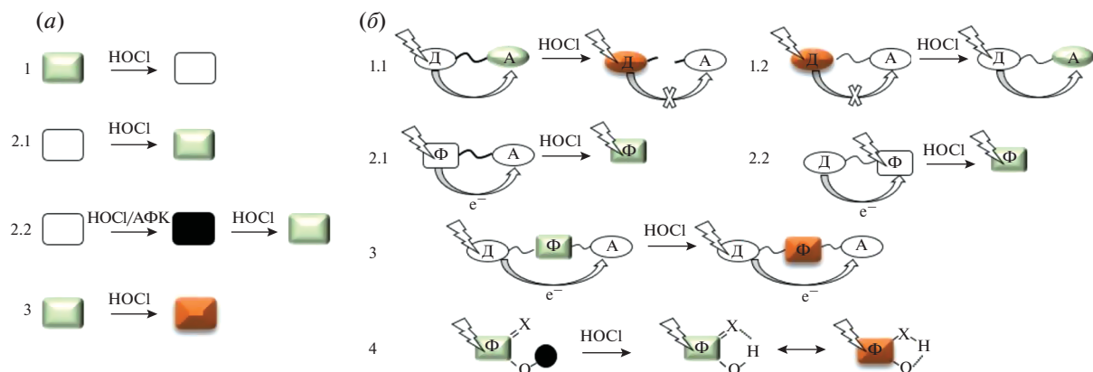
Рис. 2. Типы и механизмы флуоресцентного ответа датчиков. (а) – Общий вид типов флуоресцентного ответа: 1 – “выключения”, 2.1 – “включения”, 2.2 – “двойного замка”, 3 – “переключения”; (б) – механизмы изменения флуоресцентного ответа: 1.1 – FRET выкл, 1.2 – FRET вкл, 2.1 – а-PET, 2.2 – д-PET, 3 – ICT, 4 – ESIPT. “Ф” – флуорофор, “Д” – донор, “А” – акцептор. С изменениями и дополнениями из работы P. Gao et al. [27]. Пояснения см. в тексте.
