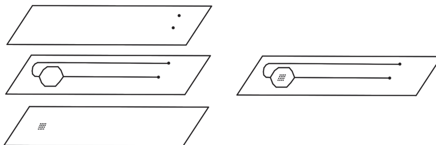
Рис. 1. Схема конструкции пленочного чипа.
