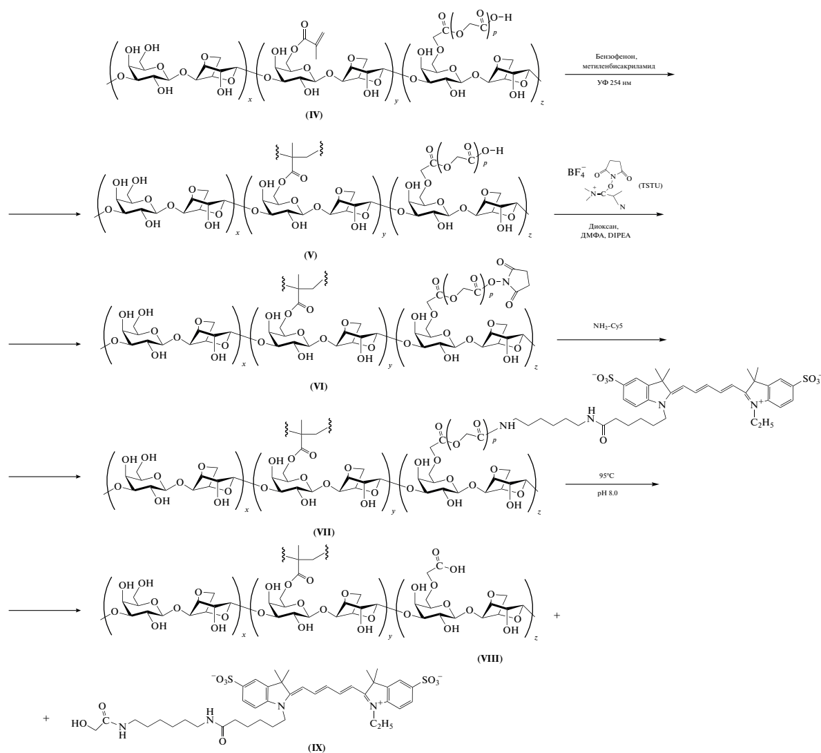
Схема 2. Кросс-сшивание и контроль метакрилкарбоксополигликолягагарозы (IV) по термоотщеплению красителя NH 2 -Cy5.
