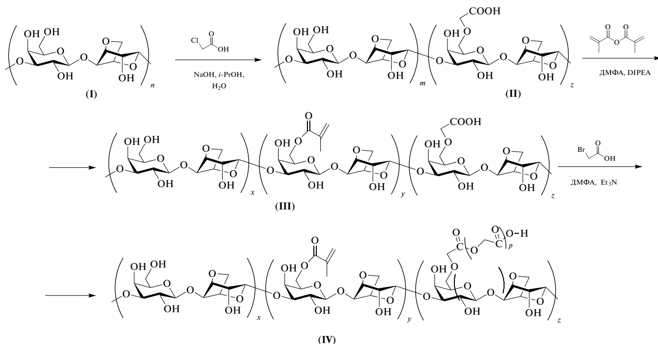
Схема 1. Получение карбоксиметилагарозы (II), метакрилкарбоксиметилагарозы (III) и метакрилкарбоксиполигликольагарозы (IV).
