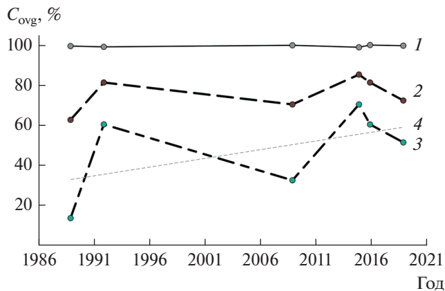
Рис. 5. Динамика степени зарастания ( C_{ovg} ) заостровного протока и мелководья “Красный ручей” в разные годы. 1 — Z_{max} , м, 2 — степень зарастания всего мелководья, 3 — степень зарастания протока, 4 — линия тренда.
