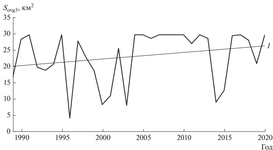
Рис. 6. Изменение площадей зарастания ( S_{ovg3} ) Волжского плеса за 31-летний период: 1 – линия тренда.
