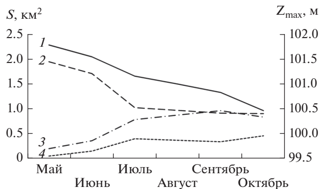
Рис. 4. Сезонная динамика площадей открытой воды ( S ) и классов макрофитов в протоке в 2016 г.: 1 – уровень воды; 2 – открытая вода; 3 – разреженные заросли; 4 – плотные заросли.
