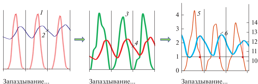
Рис. 3. Схема связи метаболизма планктона с гидрометеорологическими показателями: 1 — ФАР, \mu\text{E}/(\text{m}^2 \cdot \text{c}) ; 2 — температура воды, ^{\circ}\text{C} ; 3 — ВП; 4 — Д, \text{мг O}_2/(\text{л} \cdot \text{ч}) ; 5 — ВП/Д; 6 — содержание \text{O}_2 , \text{мг/л} . Сокращения см. рис. 1.
