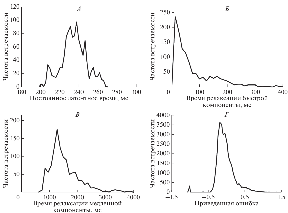
Рис. 3. Распределение параметров простой сенсомоторной реакции (ПСМР) у одного испытуемого в ходе длительного измерения. Обозначения см. рис. 2.
