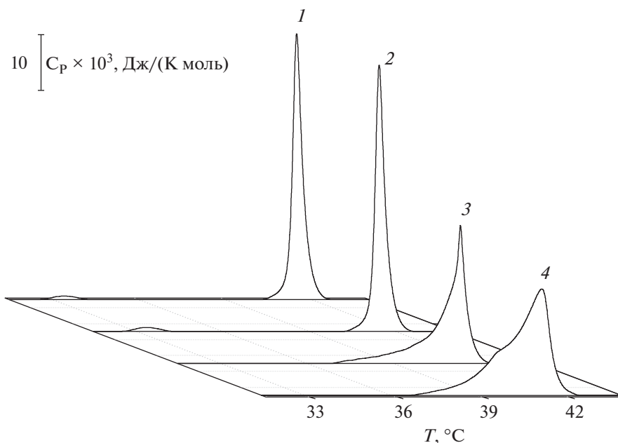
Рис. 2. Термограммы плавления ДПФХ ( C_p(T) ) в отсутствие (1) и в присутствии рутина (2), мирицетина (3) или кверцетина (4). Соотношение липид : флавонол составляет 10 : 1.
