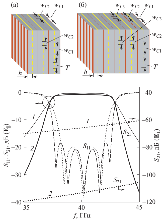
Рис. 2. Конструкции фильтров-поляризаторов третьего (а) и пятого (б) порядка, и их АЧХ соответственно – 1 и 2. Сплошные линии – при E_{||} , точки – при E_{\perp} падающей волны.
