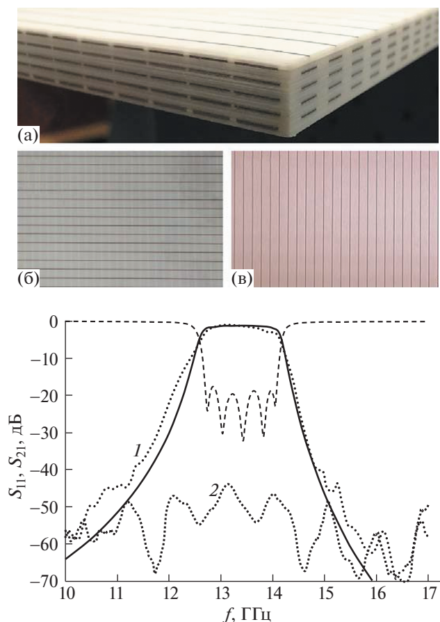
Рис. 3. Рассчитанные АЧХ фильтра-поляризатора пятого порядка при E_{\parallel} падающей волны: прямые потери – сплошная, потери на отражение – штриховая линия. Точки – измеренные характеристики прямых потерь опытного образца: 1 – при E_{\parallel} , 2 – E_{\perp} . Вверху фотография устройства (а) и фрагменты его наружных (б) и внутренних (в) решеток полосковых проводников.
