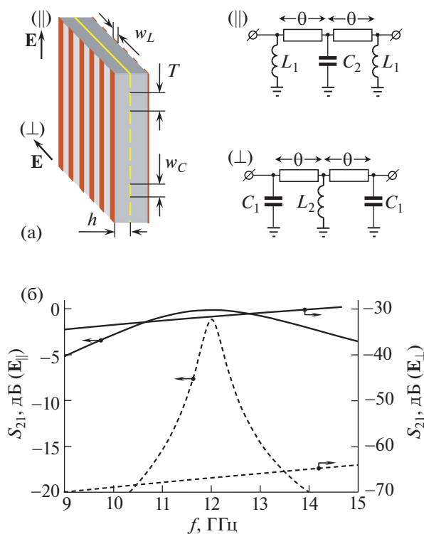
Рис. 1. а – Конструкция резонатора из двух диэлектрических слоев со скрещенными решетками полосковых проводников и его эквивалентные схемы для двух поляризаций ( E_{||} и E_{\perp} ) падающей электромагнитной волны, б – частотные зависимости прямых потерь резонаторов.
