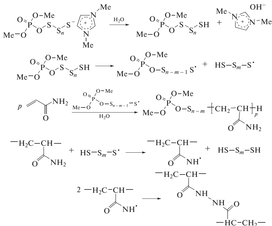
Схема 12. Синтез шитого полиакриламида в присутствии (фосфоноокси)олигосульфанида 1,3-диметилимидазолия [146].
