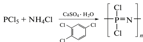
Схема 2. Синтез [-N\text{P}(\text{Cl})_2-]_n из пентахлорида фосфора и хлорида аммония [50].
