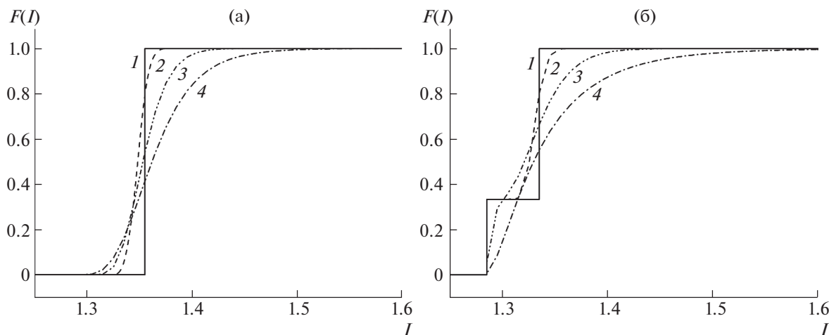
Рис. 4. Эмпирические функции распределения (16) индекса I_{VS} при различных значениях параметра \varepsilon : а) триангуляция на основе базового параллелепипеда куба ( 1 - \varepsilon = 0, 2 - \varepsilon = 0.05, 3 - \varepsilon = 0.15, 4 - \varepsilon = 0.235 ); б) триангуляция на основе базового параллелепипеда ромбоэдра ( 1 - \varepsilon = 0, 2 - \varepsilon = 0.05, 3 - \varepsilon = 0.15, 4 - \varepsilon = 0.272 ).
