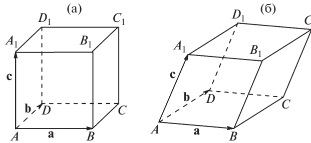
Рис. 3. Базовый параллелепипед модельной триангуляции: базисные вектора a , b , c имеют единичную длину, начинаются в точке A и заканчиваются в точках B , D и A 1 соответственно: а) куб (базисные вектора ортогональны друг другу); б) ромбоэдр (базисные вектора попарно составляют друг с другом угол \pi/3 ).
