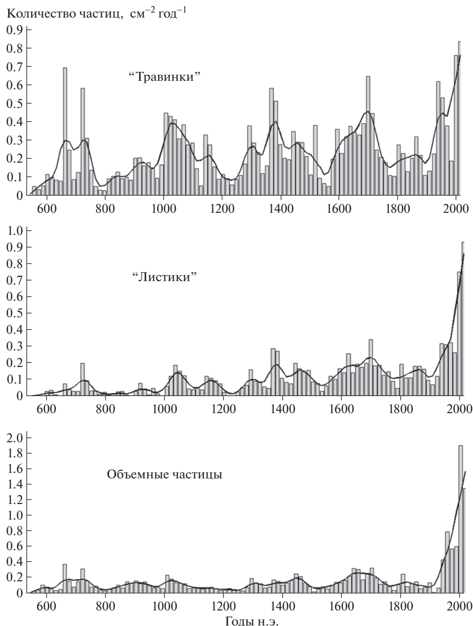
Рис. 1. Скорость накопления углистых частиц в донных отложениях озера Ширы.
