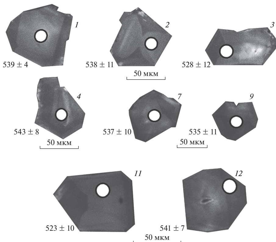
Рис. 4. Микрофотографии кристаллов циркона из плагиигранитов Тектурмасской зоны, выполненные на электронном микроскопе Camscan MX 2500S в режиме катодоллюминесценции (проба ТЕК-2202). Номера точек соответствуют номерам в табл. 1.
