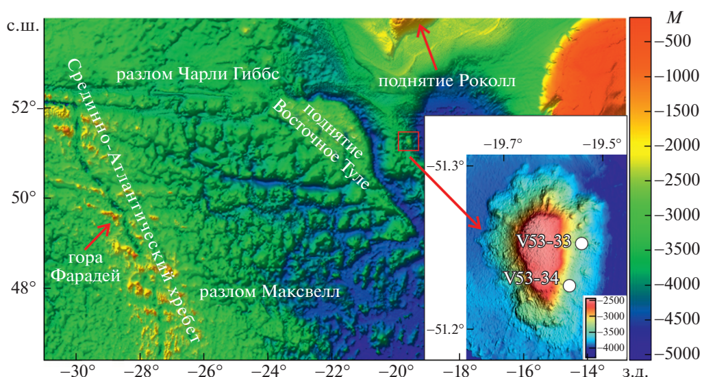
Рис. 1. Строение океанического дна между разломами Максвелл и Чарли Гиббс (на основе карты GEBCO [2]). Положение подводной горы 51—19 обведено красным квадратом. Справа дана шкала глубин. На врезке даны батиметрическая карта подводной горы и положение станций драгирования из работы [3], в нижнем правом углу врезки — шкала глубин в метрах.
