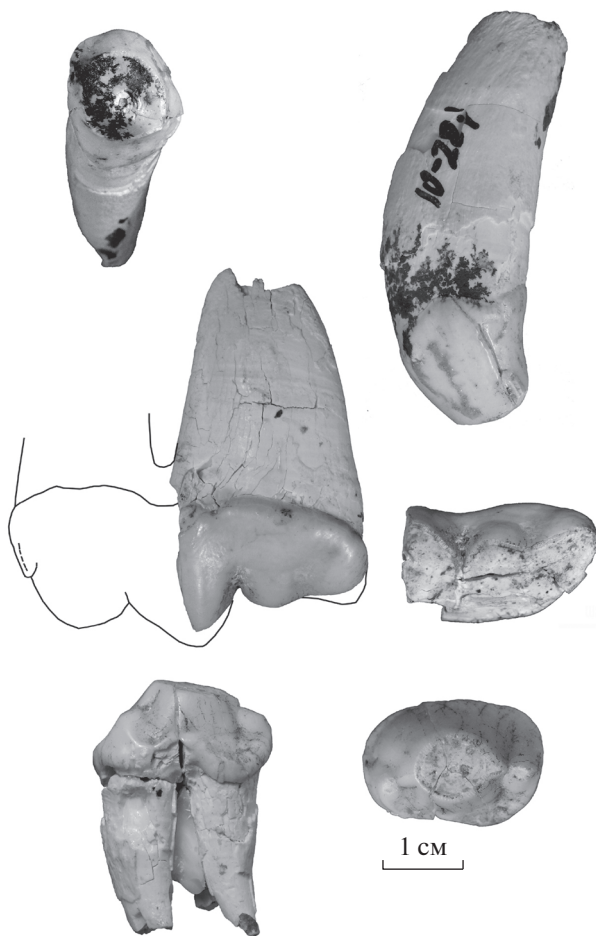
Рис. 1. Pachycrocuta brevirostris (Gervais, 1850): экз. ПИН, № 5644/83, левый I3 с окклюзиальной (вверху слева) и буккальной (вверху справа) сторон; экз. ПИН, № 5644/79, фрагмент левого P4 с лабиальной (в середине слева, прорисованы реконструированные контуры зуба) и окклюзиальной (в середине справа) сторон; экз. ПИН, № 5644/81, правый p2 с лингвальной (внизу слева) и окклюзиальной (внизу справа) сторон; Крым, пещера Таврида; нижний плейстоцен.
