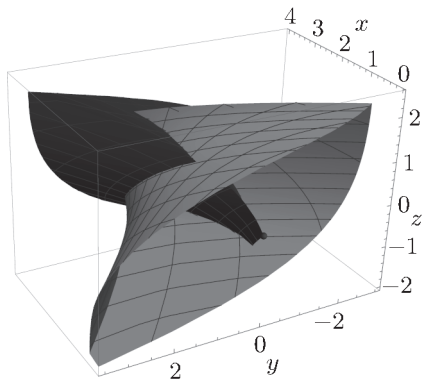
Рис. 6. Группа \operatorname{SE}(2) .
