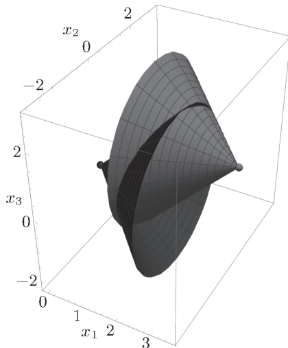
Рис. 1. Пространство Минковского.
