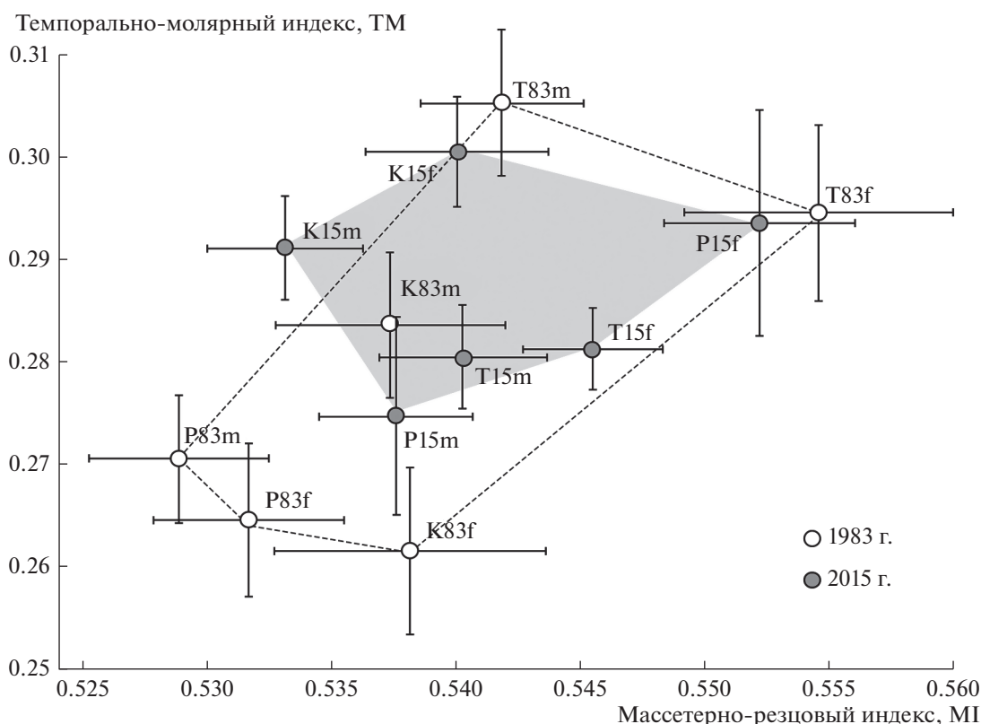
Рис. 4. Сравнение средних значений морфофункциональных мандибулярных индексов МI и ТМ с учетом стандартных ошибок ( \pm SE ) в выборках самцов (m) и самок (f) тоцкой (Т), платовской (Р) и сакмарской (К) популяций рыжей полевки разных лет (83 – 1983 г. и 15 – 2015 г.).
