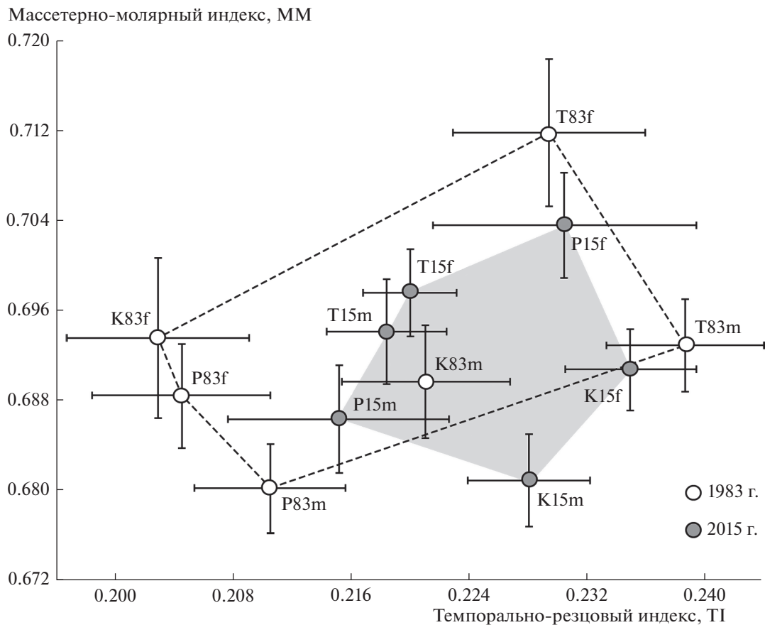
Рис. 5. Сравнение средних значений морфофункциональных мандибулярных индексов ТI и ММ с учетом стандартных ошибок ( \pm SE) в выборках самцов (m) и самок (f) тоцкой (Т), платовской (P) и сакмарской (К) популяций рыжей полевки разных лет (83 – 1983 г. и 15 – 2015 г.).
