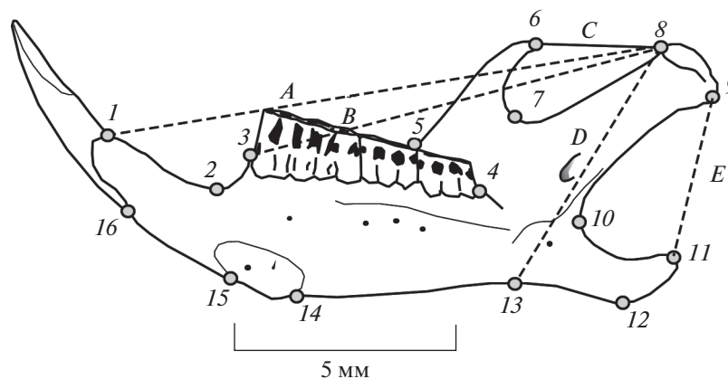
Рис. 1. Схема размещения на лингвальной стороне нижнечелюстной ветви рыжей полевки 16 меток-ландмарков (1–16) и промеров (A–E), необходимых для вычисления мандибулярных функциональных индексов: TI, TM, MI, MM, AM (формулы для их расчета см. в тексте).
