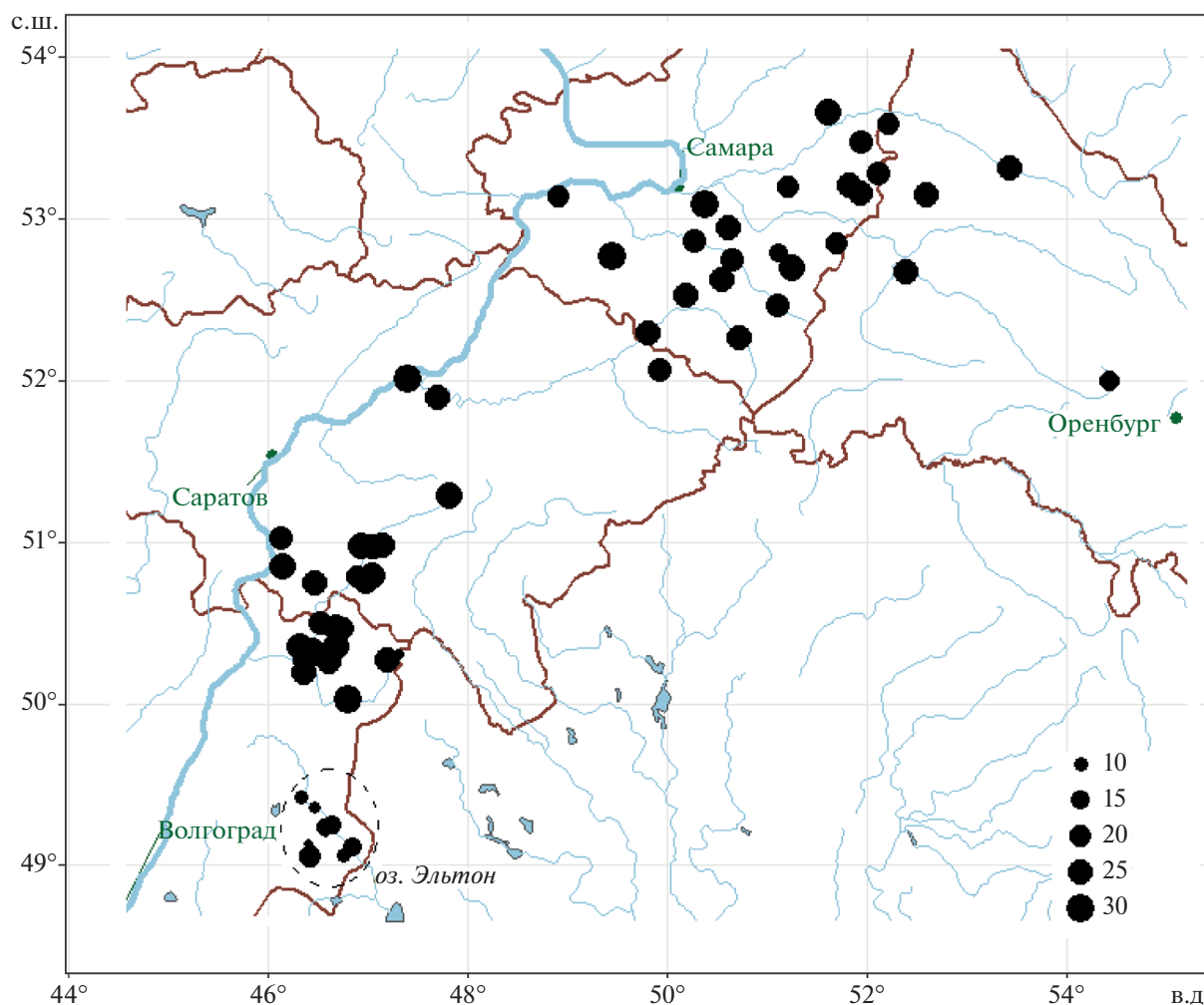
Рис. 1. Территория проведения исследований; диаметр кружков в районах гидробиологической съемки пропорционален квадратичной энтропии Рао донных сообществ.
