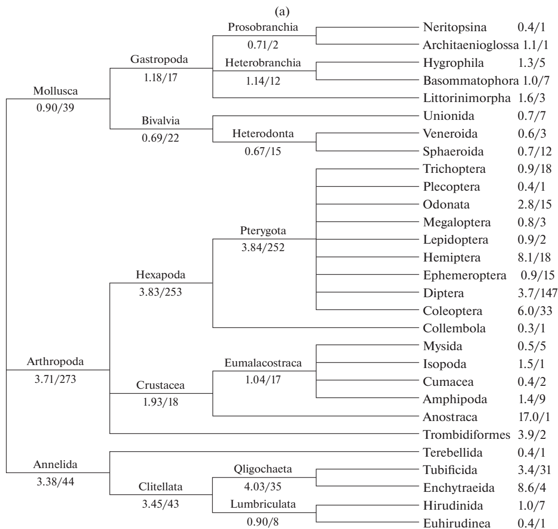
Рис. 3. Кладогаммы таксономического состава макрозообентоса по результатам исследования (средняя соленостная толерантность/число видов в кладе): а — общее дерево от Phylum до Order; б — фрагмент дерева для Diptera, Chironomidae от SubFamily до Genus.
