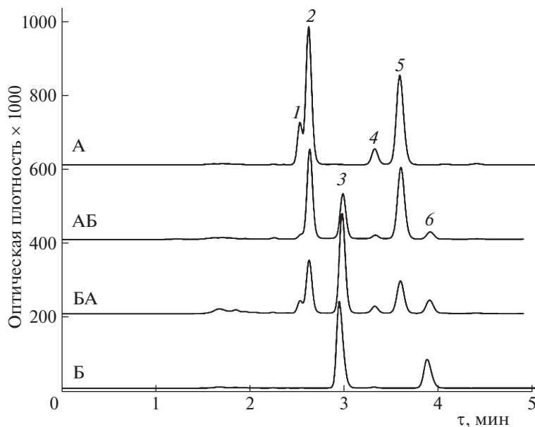
Рис. 1. Разделение антоцианов плодов черной смородины (а) и аронии Мичурина (б). Колонка 4.6 \times 150 Symmetry C18, 3.5 \mu\text{m} ; подвижная фаза: 10 об. % муравьиной кислоты и 10 об. % ацетонитрила в воде, 0.8 мл/мин. Температура термостата колонки 40^\circ\text{C} . Составы маточных растворов над глинами после сорбции антоцианов – описание АБ и БА – см. в тексте. Антоцианы: 1 – Dp3Glu, 2 – Dp3Rut, 3 – Cy3Gala, 4 – Cy-3-Glu, 5 – Cy3Rut.
