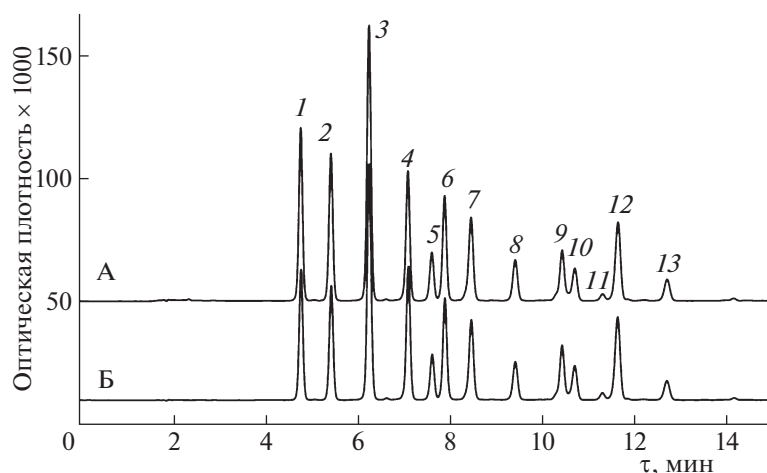
Рис. 2. Разделение антоцианов плодов черники после очистки на патронах С18 (А) и на бентонитовой глине (Б). Хромотографические условия см. рис. 1, нумерацию пиков см. табл. 1.
