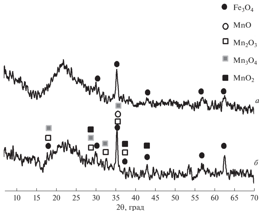
Рис. 1. Рентгенограммы НПС-матрицы (а) и композита, синтезированного на ее основе (б).
