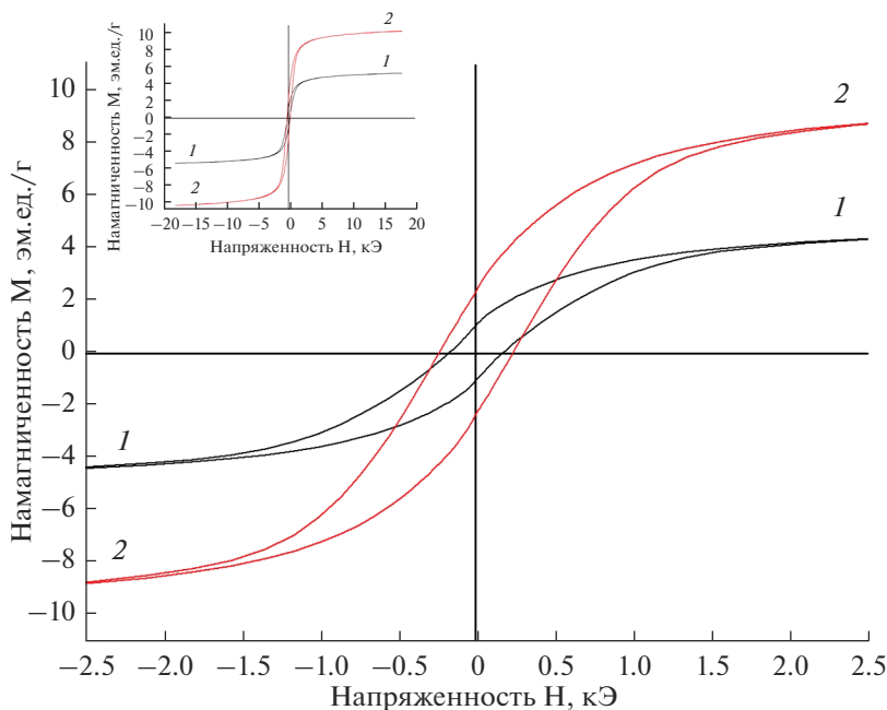
Рис. 3. Зависимости намагниченности НПС-матрицы (1) и композита (2), синтезированного на ее основе, от приложенного магнитного поля до 2.5 кЭ и до 18 кЭ (на врезке) при 293 К.
