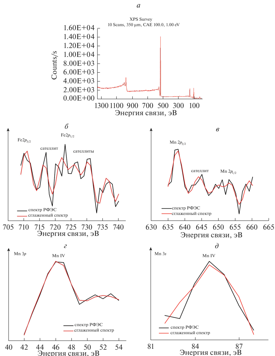
Рис. 2. Обзорный РФЭС спектр ( a ) и фотоэлектронные спектры Fe 2 p ( b ), Mn 2 p ( в ), Mn 3 p ( г ), Mn 3 s ( д ) синтезированного композита, снятые при 293 К.
