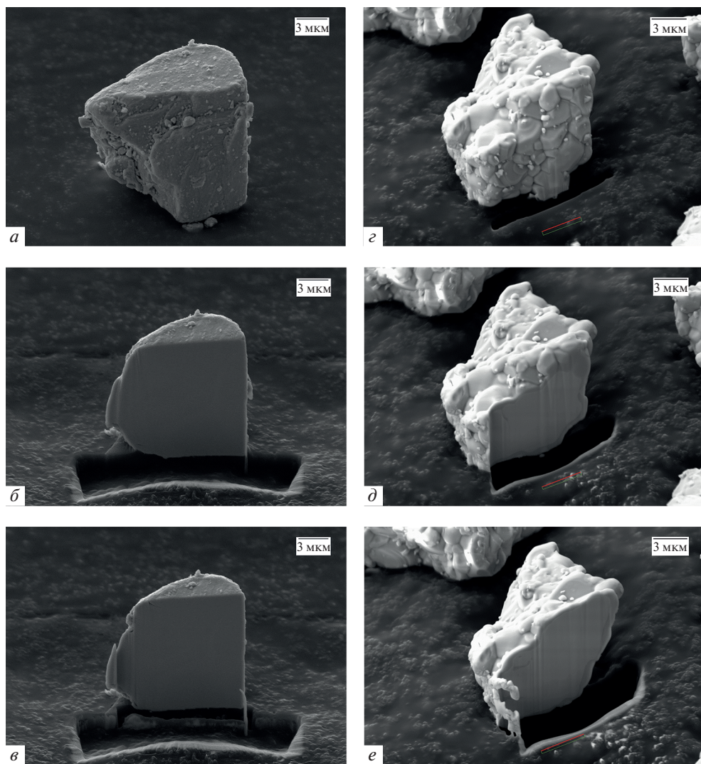
Рис. 3. Микрофотографии послойно стравленных слоев ионами \text{Ga}^+ исходной ( а, б, в ) и окисленной ( z, д, е ) частиц n -PbSe.
