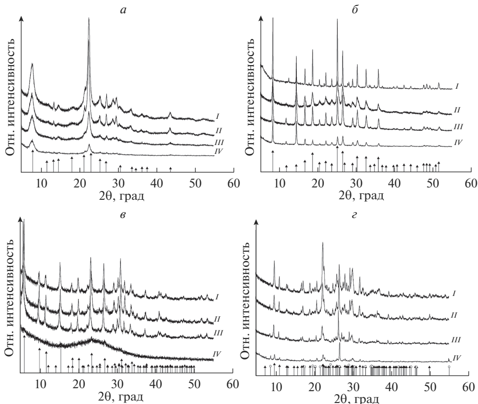
Рис. 1. Рентгеновские дифрактограммы образцов цеолитов, обработанных в модельных биологических средах в течение 7 сут: H-Beta ( a ), H-Rho ( б ), H-Y ( в ), КЛ ( з ). ▲ — штрих-диаграммы стандартов цеолитов Beta, Rho, Y, K; ○ — иллит. I — исходный цеолит, II — цеолит, обработанный в среде с pH 6.9, III — цеолит, обработанный в среде с pH 8, IV — цеолит, обработанный в среде с pH 1.8.
